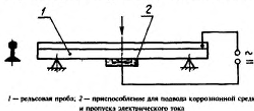
Рисунок 2 — Схема испытания рельсовых проб на коррозионную усталость
