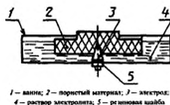
Рисунок 1 — Приспособление для подвода коррозионной среды и пропуска электрического тока через зону контакта подошвы рельса со средой в процессе коррозионно-усталостных испытаний
