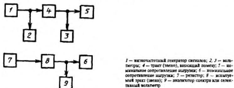
Рисунок 6 — Структурная схема измерения защищенности максимального сигнала от выятной переходной помехи
