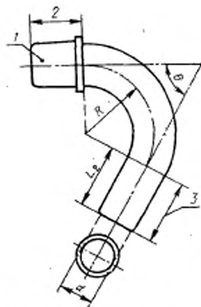
1—охватываемая деталь конического соединения номинальным диаметром 15 мм по ГОСТ Р 50327.1; 2—сторона аппарата; 3—сторона пациента.
