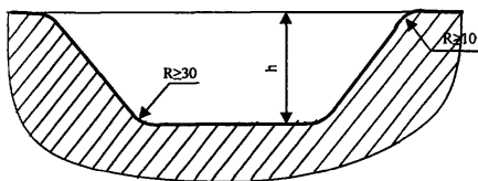
Рисунок 6.1- Вид поперечное сечение подготовленной под заварку выборки с радиусными переходами
