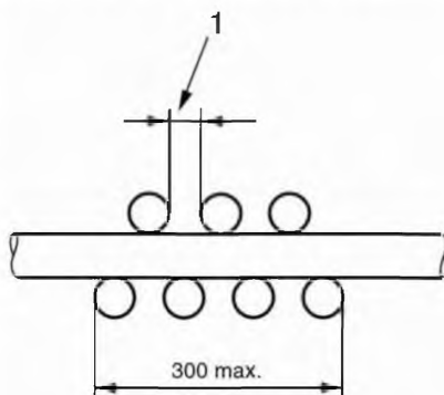
Рисунок 1 – Типичное расположение с зазором отрезков кабеля, закрепленных на обеих сторонах стандартной лестницы (категория A F/R)
