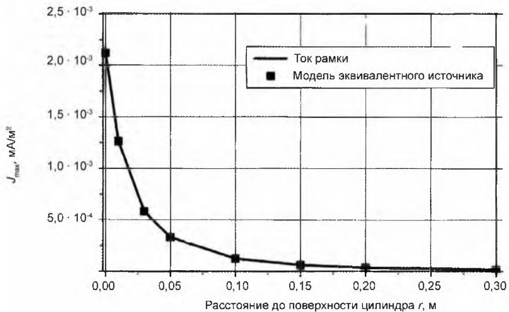
Рисунок F.5 – Зависимость максимальной плотности тока J_{\max} от расстояния
