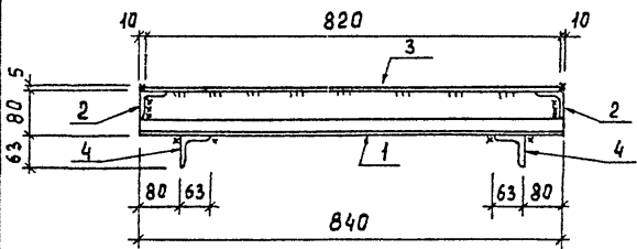
РАЗРЕЗ 1-1
