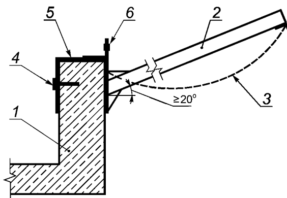
1 — стена (подоконник); 2 — опора из труб; 3 — сетка; 4 — анкеры для прикрепления устройства 5 к стене; 5 — устройство для прикрепления опоры к стене; 6 — место прикрепления опоры к устройству 5
