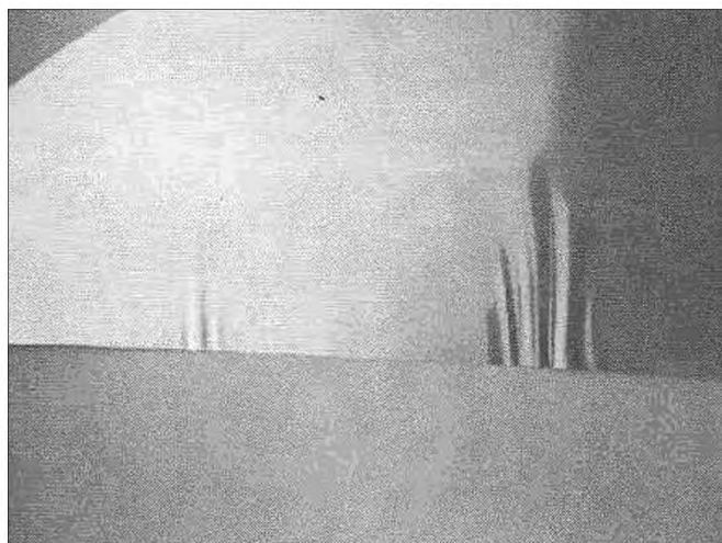
Рисунок А.61 — Местное замятие кромки (жеванность)
