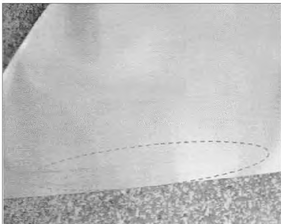
Рисунок А.67 — Темные полосы прокатного происхождения
