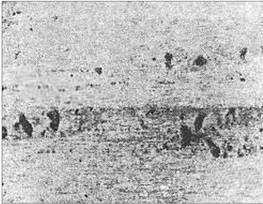
Рисунок А.12 — Закаты неметаллического материала
