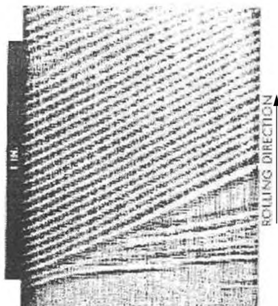
Рисунок А.19 — Линии скольжения (Людерса)
