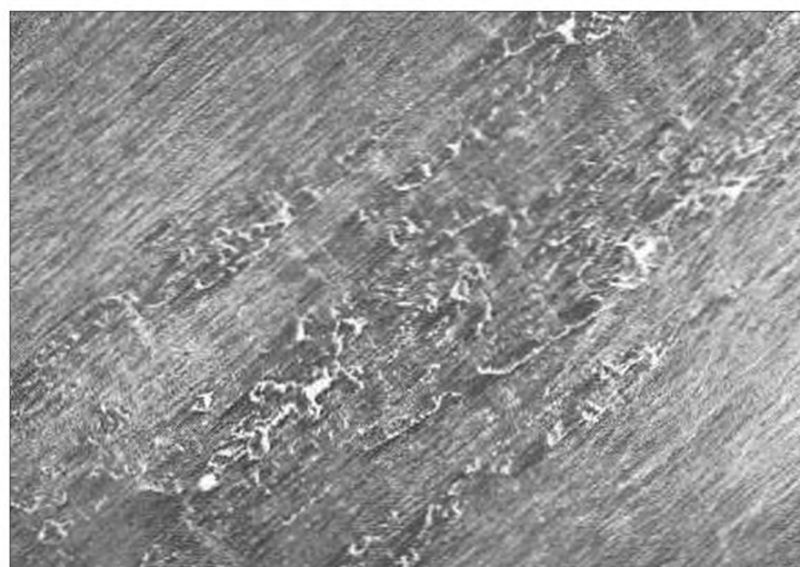
Рисунок А.68 — Привар витков
