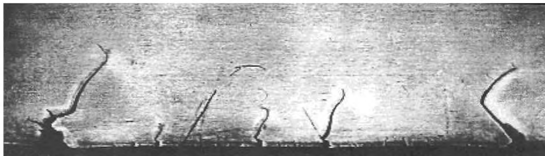
Рисунок А.17 — Рваная кромка
