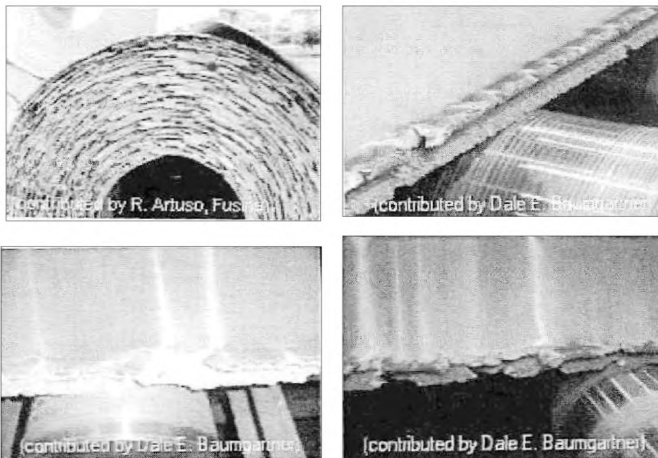
Рисунок А.8 — Трещины по кромке
