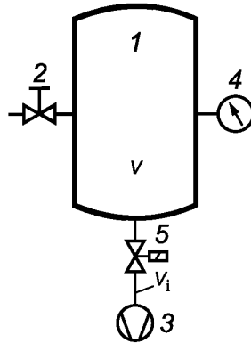
1 — измерительная камера; 2 — клапан напуска газа; 3 — испытываемый насос; 4 — вакуумметр для измерения p_{t1} , p_{t2} , p_{t3} ; 5 — быстродействующий клапан; V — объем измерительной камеры; V_i — объем трубопровода между испытываемым насосом и быстродействующим клапаном
