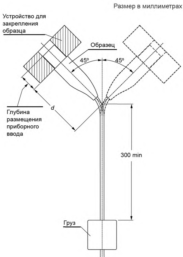
Рисунок 2 — Устройство для испытания на изгиб
