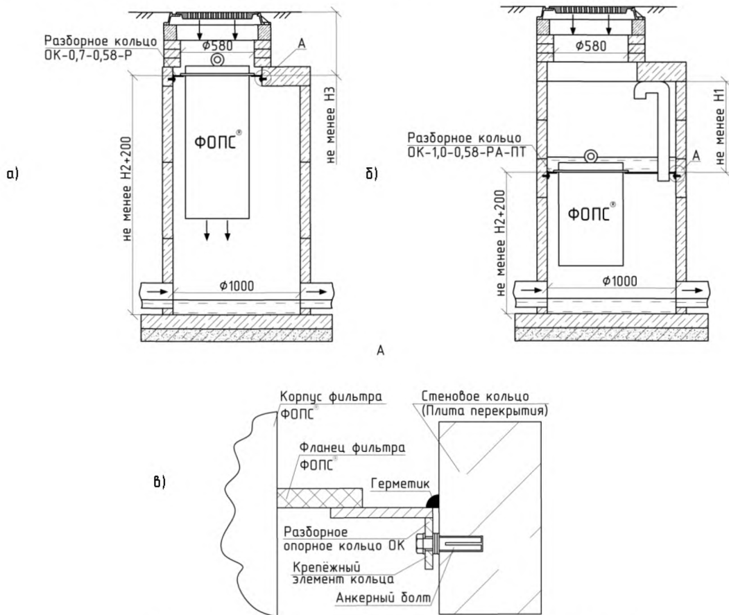
Рис. 1. Схемы установки фильтров ФОПС® на разборные кольца ОК: а - на кольцо ОК-0,7-0,58-Р; б - на кольцо ОК-1,0-0,58-РА-ПТ; в - крепление опорного кольца в горловине плиты перекрытия.
