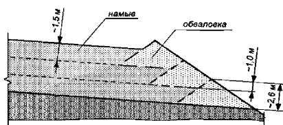
Рисунок 2.7 — Дамбы вторичного обвалования ([40])
