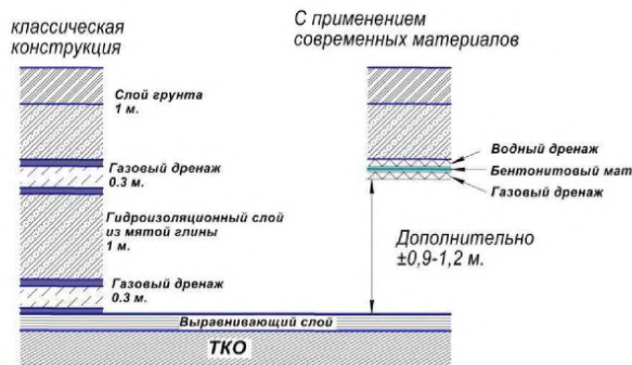
Рисунок 2.4 — Конструкция ПФЭ с использованием бентонитового мата ([28])
