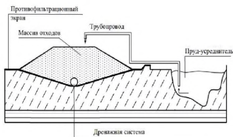
Рис. 2.17 — Схема рециркуляции фильтрационных вод ([55]) (ОРО ТКО в Пермском крае)
