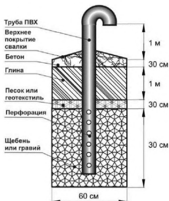
Рис. 2.13 — Газорыпуск при устройстве траншейной системы сбора биогаза ([46])
