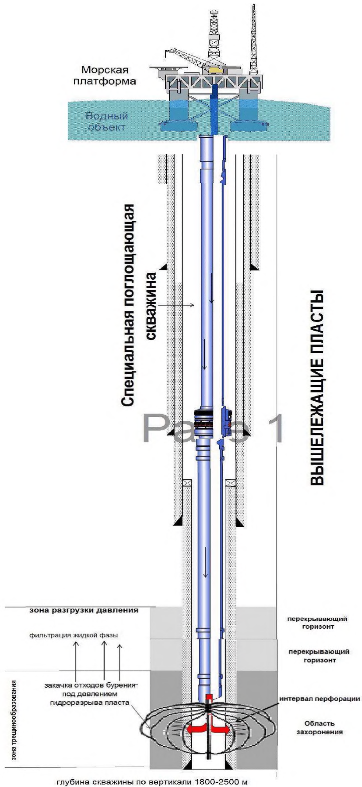
Рисунок 2.9 — Схема обустройства специальной поглощающей скважины (Сахалинская область) ([44])
