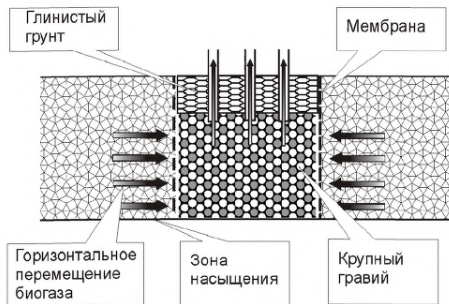
Рис. 2.11 — Устройство горизонтальной траншеи ([47])
