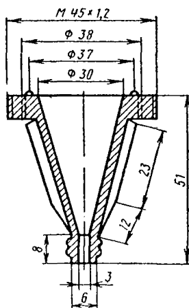
Рис. 4. Плексигласовый патрон для фильтров
