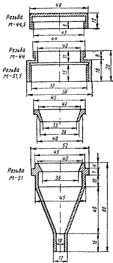
Рис. 1. Металлический патрон для фильтров
