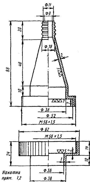
Рис. 2. Металлический патрон, применяемый с кассетой
