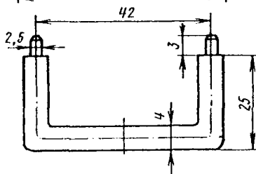
Рис. 3. Металлическая кассета для закрепления фильтров
