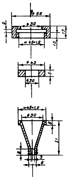
Рис. 2. Плексигласовый патрон для фильтра
