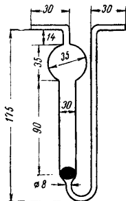
Рис. 8. Погло- тительный прибор с пористой пластин- кой.
