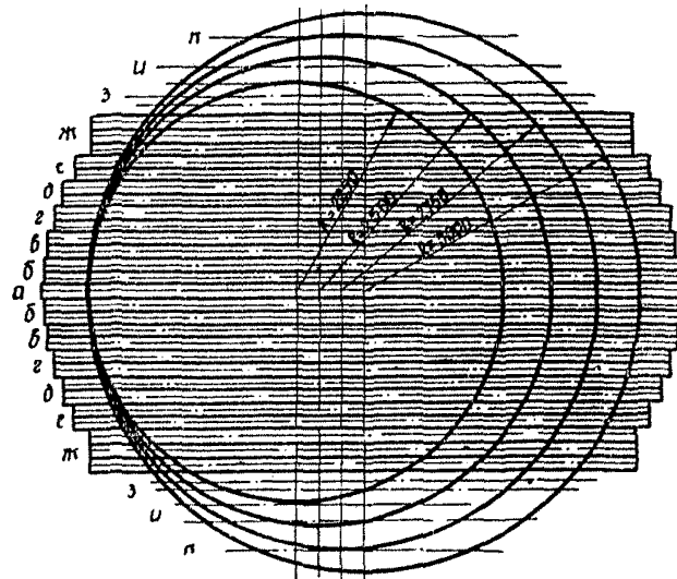
Схема расположения балок под предохранительным щеликом
