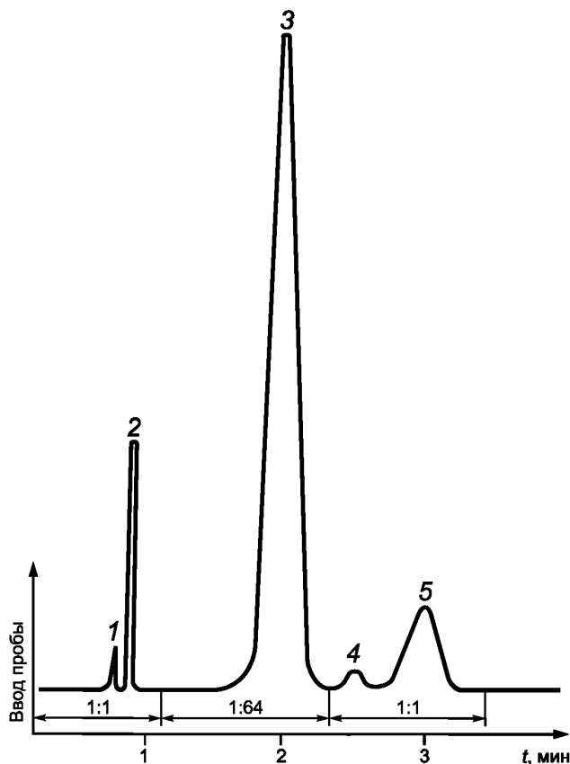
Рисунок 1 — Типовая хроматограмма технического фурфурола
