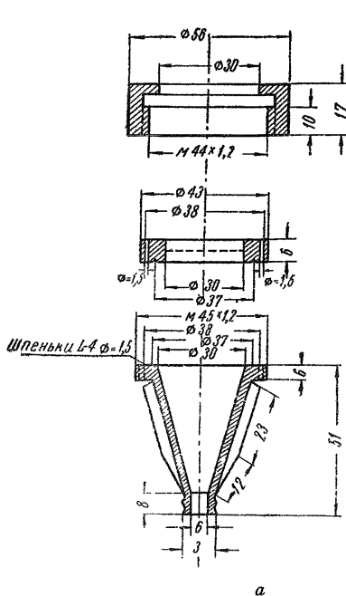
Рис. 3. Патрон плексигласовый для бумажного и других фильтров.
