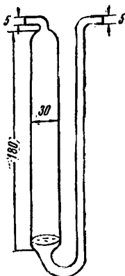
Рис. 1. Поглотительный прибор с пористой пластинкой.
