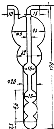
Рис. 2. Поглотительный прибор Рыхтера.
