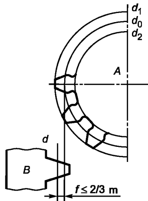
A — шестерня; B — рейка; d_1 — диаметр окружности вершин зубьев шестерни; d_0 — диаметр делительной окружности шестерни; d_2 — диаметр окружности впадин зубьев шестерни; d — делительная прямая рейки; e — не более 1/3 модуля; f — не более 2/3 модуля
