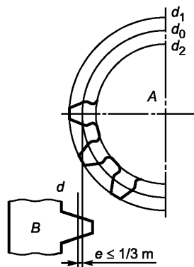
Рисунок 9 — Нормальное зацепление зуба шестерни
