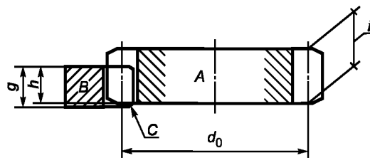
A — шестерня; B — рейка; C — фаска; d_0 — диаметр делительной окружности шестерни; g — длина зуба; h — 90 % от длины зуба; i — длина зуба шестерни по d_0
