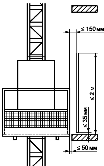
Рисунок 5 — Пример дверей погрузочной площадки в полную высоту
