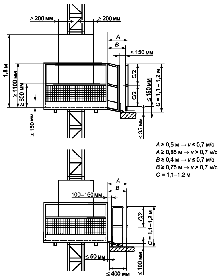
Рисунок 6 — Пример дверей погрузочной площадки уменьшенной высоты
