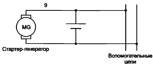
Рисунок А.6 — Система электропитания автономного железнодорожного подвижного состава с генераторами переменного тока, выпрямителями, преобразователем частоты и тяговым двигателем постоянного тока
