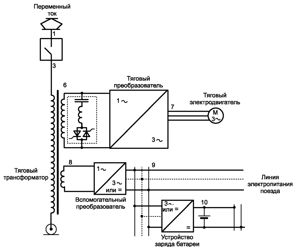
Рисунок А.2 — Система электропитания железнодорожного подвижного состава переменного тока с тяговым преобразователем и электродвигателем переменного тока, оснащенная компенсатором реактивной мощности
