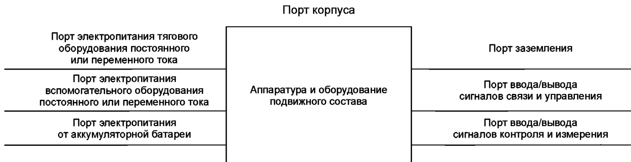
Рисунок 1 — Основные типы портов
