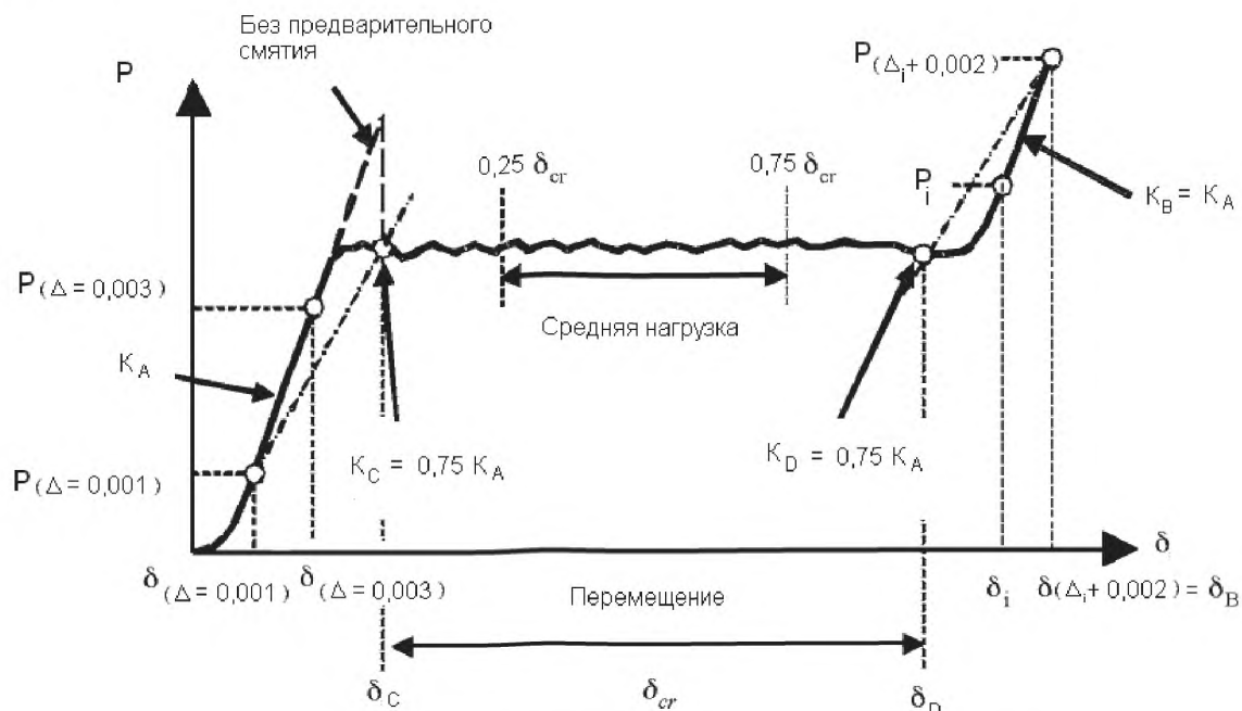
P — нагрузка; P_{(\Delta=0,003)} — нагрузка при \delta_{(\Delta=0,003)} ; P_{(\Delta=0,001)} — нагрузка при \delta_{(\Delta=0,001)} ; K_A — угол наклона начального линейного участка графика; K_B — угол наклона конечного линейного участка графика; K_C — угол наклона прямой до начала смятия образца; K_D — угол наклона прямой после смятия; P_{(\Delta_i+0,002)} — нагрузка при \delta_{(\Delta_i+0,002)} ; P_i — нагрузка при \delta_i ; \delta — перемещение; \delta_{(\Delta=0,001)} — перемещение активного захвата, при котором \Delta стремится к 0,001; \delta_{(\Delta=0,003)} — перемещение активного захвата, при котором \Delta стремится к 0,003; \delta_c — перемещения активного захвата, когда началось разрушение образца; \delta_D — перемещения активного захвата, когда закончилось смятие образца; \delta_{cr} — перемещение активного захвата во время смятия; \delta_i — перемещение активного захвата в точке i перед смятием; \delta_{(\Delta_i+0,002)} — перемещение активного захвата после смятия образца, при котором \Delta на 0,002 больше \delta_i Рисунок 6 — Определения, описывающие отношение усилия сжатия материала среднего слоя многослойных конструкций к смещению/отклонению
