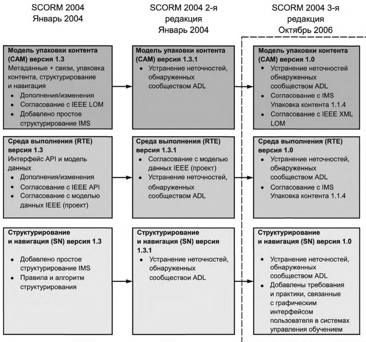
Рисунок 2 — Эволюция SCORM 2004
