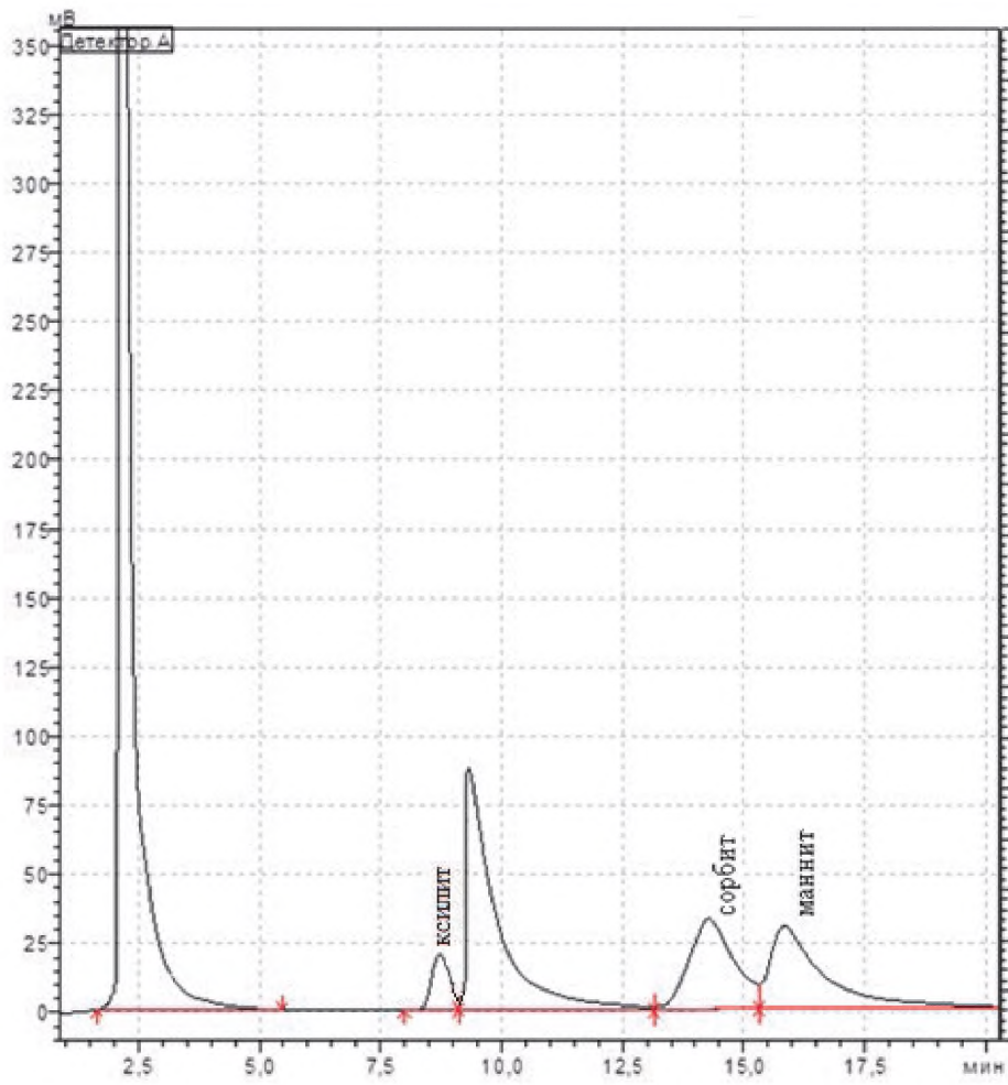
Рисунок Б.2 — Пример хроматограммы яблочного сока с добавкой стандартного раствора ксилита, сорбита, маннита с концентрациями соединений по 5 мг/см 3
