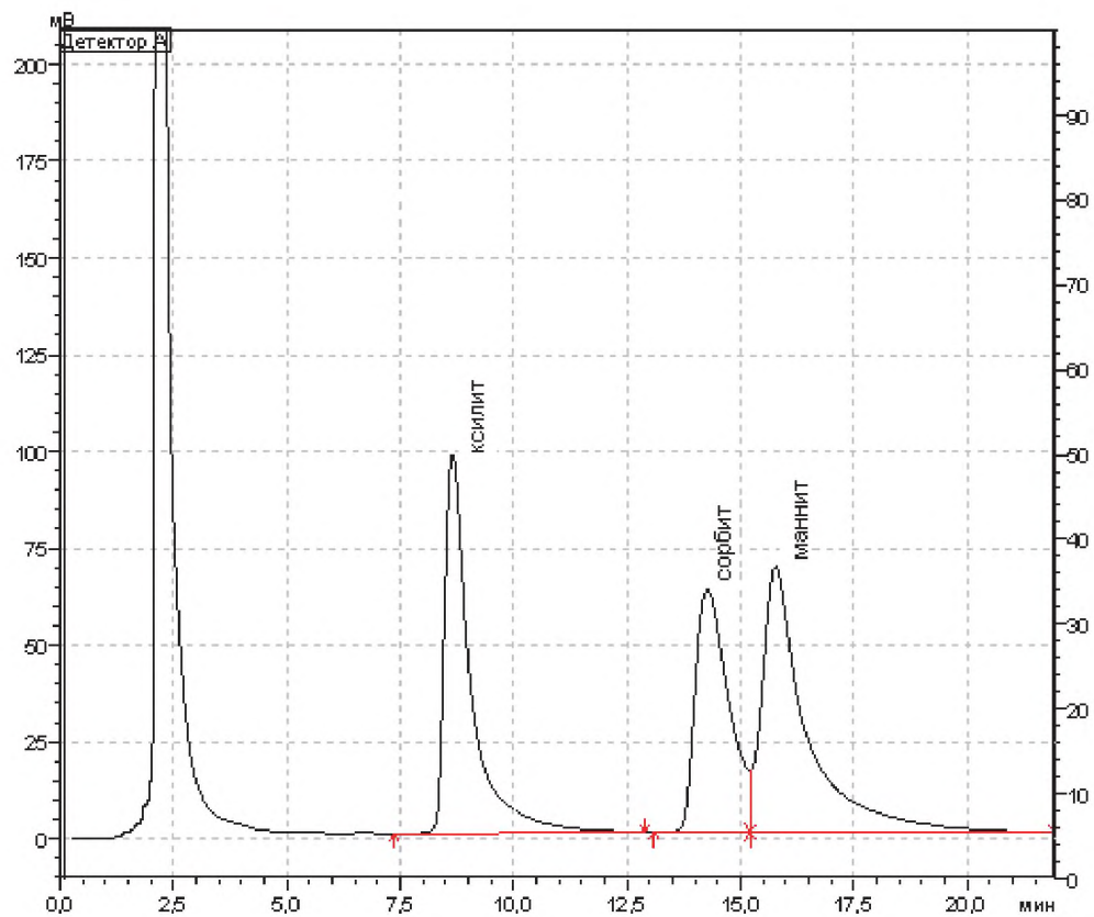
Рисунок Б.3 — Пример хроматограммы стандартного раствора ксилита, сорбита, маннита в воде с концентрациями соединений в растворе по 50 мг/см 3
