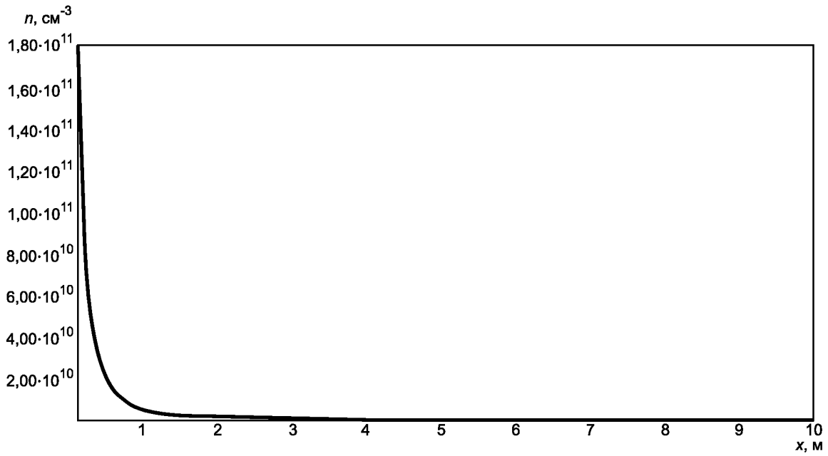
Рисунок Б.7 — Распределение концентрации плазмы n , \text{cm}^{-3} , в струе двигателя СПД-70 вдоль оси струи
