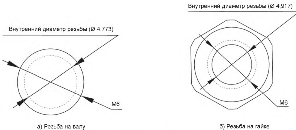
Рисунок 2 — Примеры ЭМД с резьбой М6 согласно ГОСТ 24705
