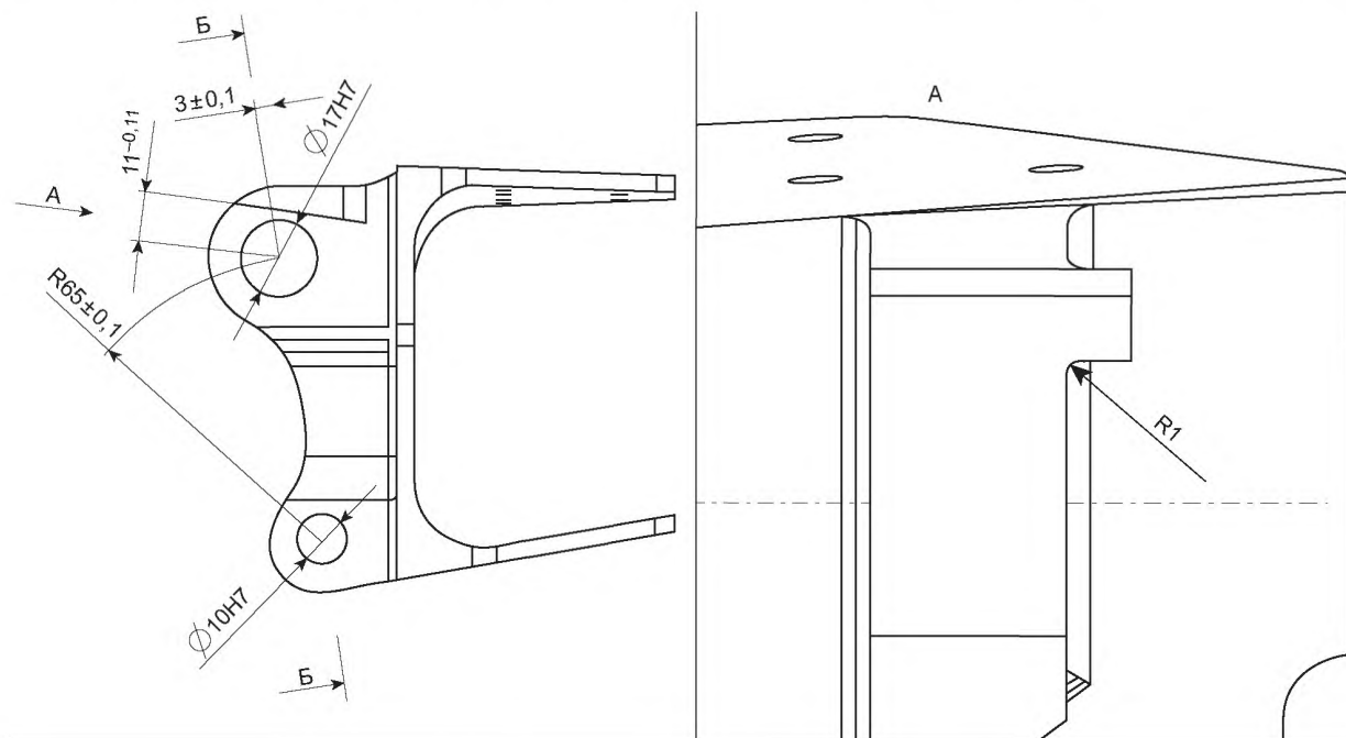
Рисунок В.1 — Пример выполнения дополнительного вида
