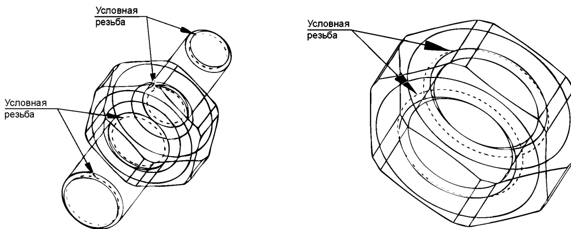
а) Обозначение резьбы на шпильке
