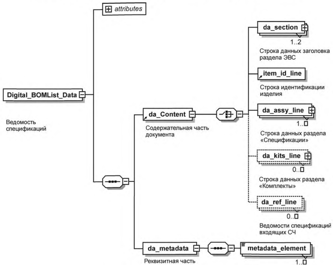
Рисунок В.1— Логическая модель данных электронной ведомости спецификаций
