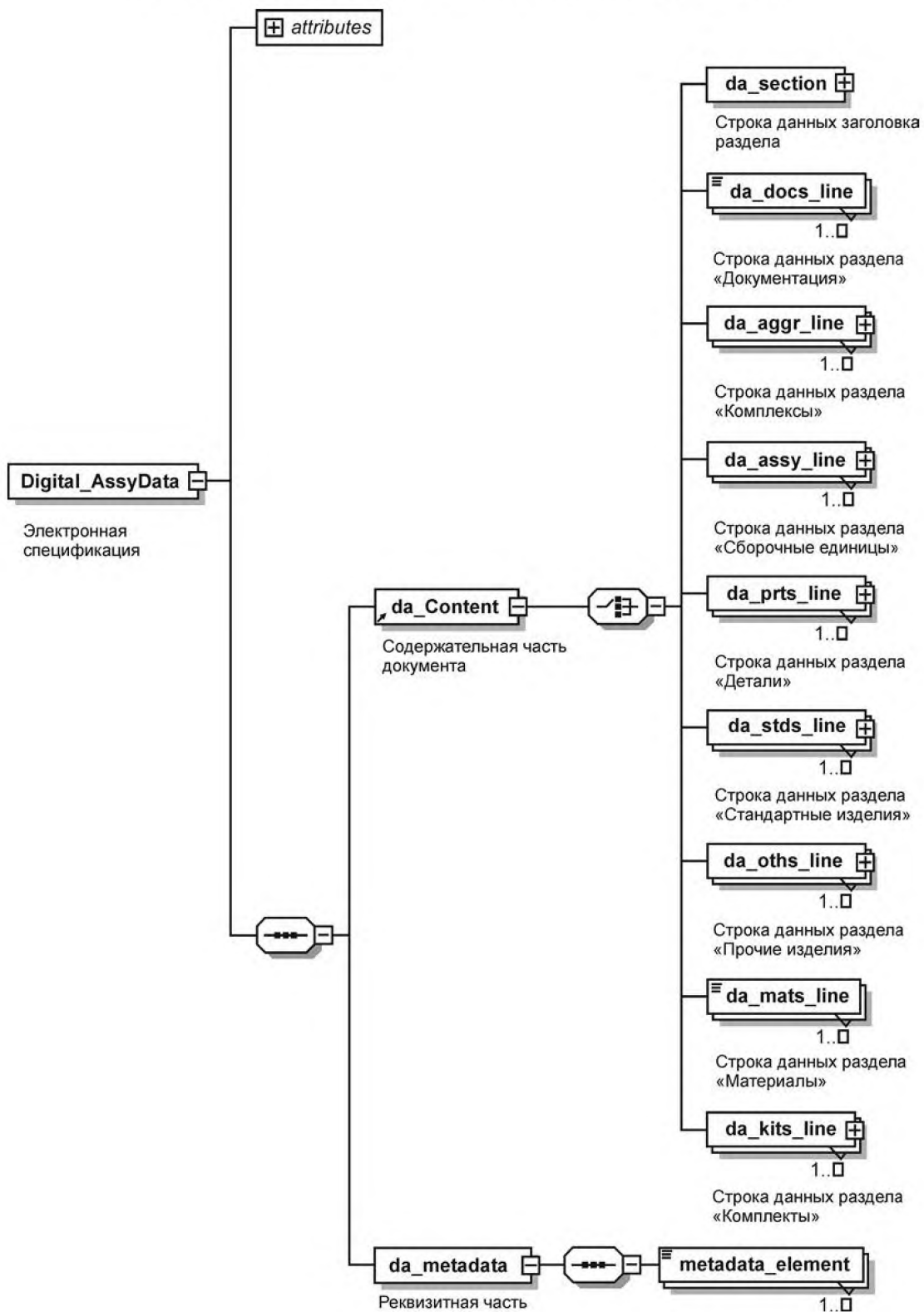
Рисунок Б.1 — Логическая модель данных электронной спецификации
