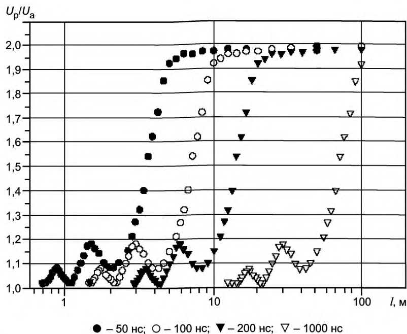
Рисунок 4 — Максимальное увеличение напряжения на зажимах машины в функции длины кабеля l и различного времени нарастания импульса для двухуровневого преобразователя
