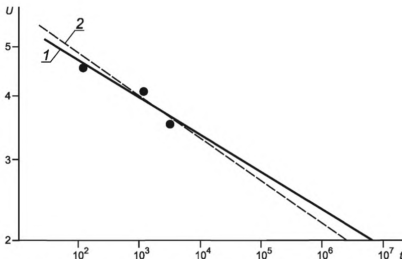
1 — срок службы межвитковой изоляции; 2 — срок службы корпусной изоляции; t — время до пробоя; U = U_{испыт}/U_{lim} — для витковой изоляции; U = U_{испыт}/U_{ном} — для корпусной изоляции
