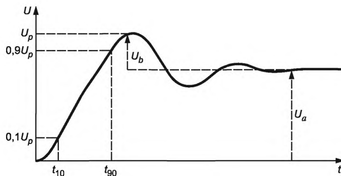
Рисунок 1 — Параметры импульса напряжения
