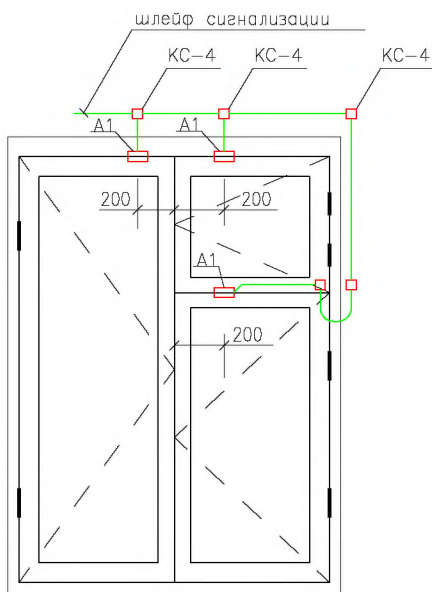
Схема блокировки окна
