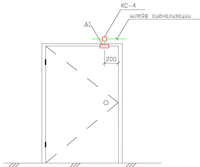
Схема блокировки двери
