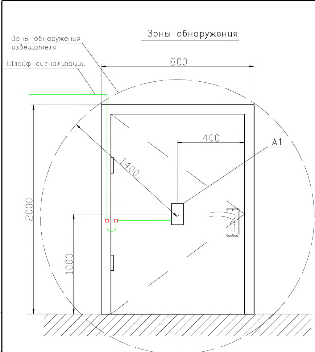
A1– Извещатель охранный поверхностный вибрационный .
