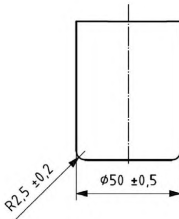
Рисунок 1 – Схема штампа
