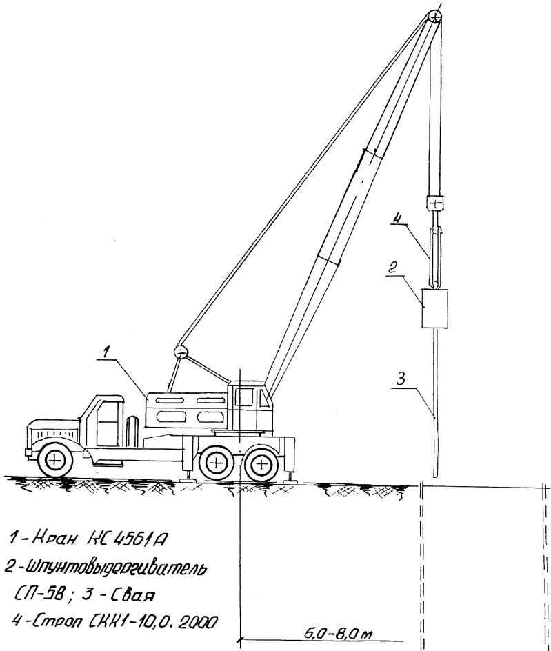
Рис. 4-1. Извлечение шпунта
