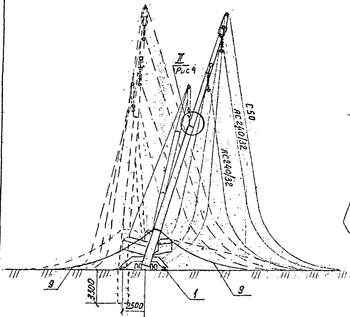
Рис.3 Узел I
