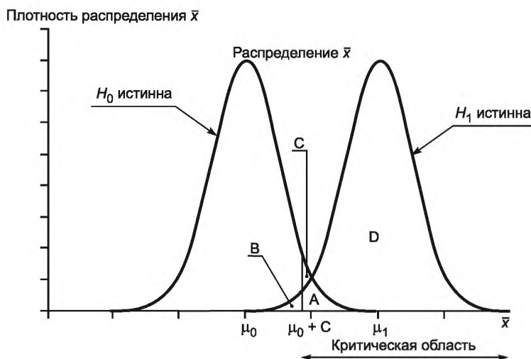
Рисунок 1 — Односторонний критерий
