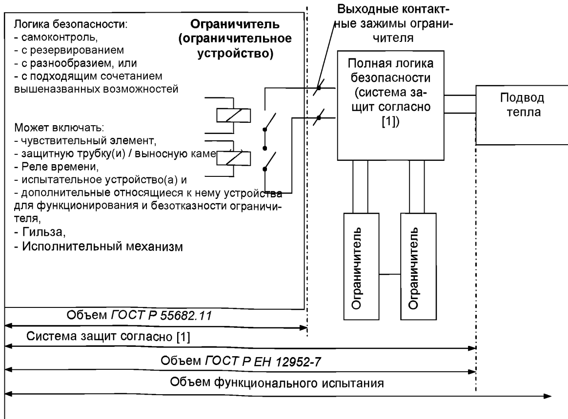
Рисунок А.1 – Ограничительное устройство
