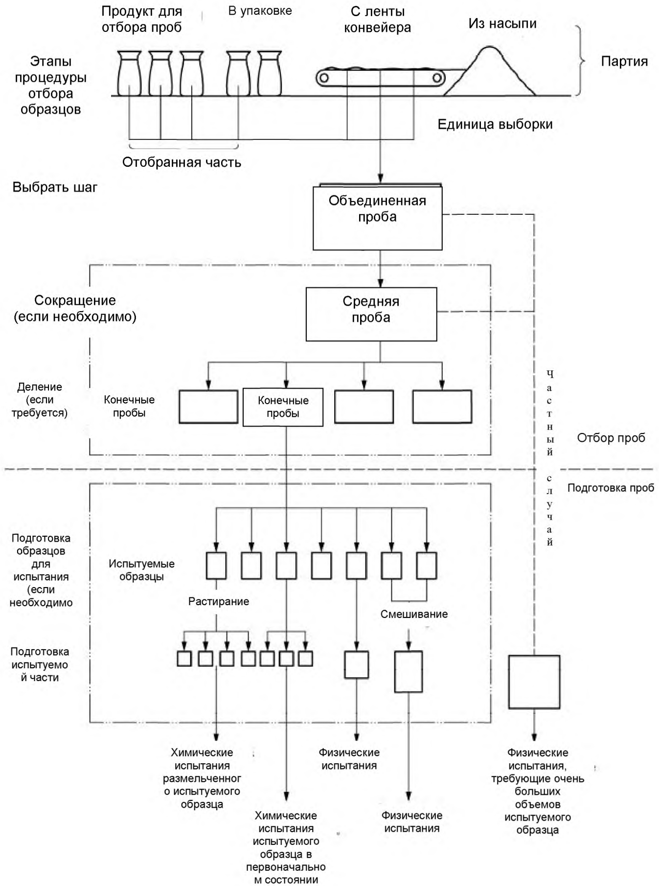
Рисунок 1 — Схема отбора проб твердых веществ
