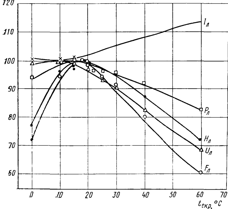
Зависимость параметров люминесцентных ламп мощностью 30 Вт от температуры окружающей среды
