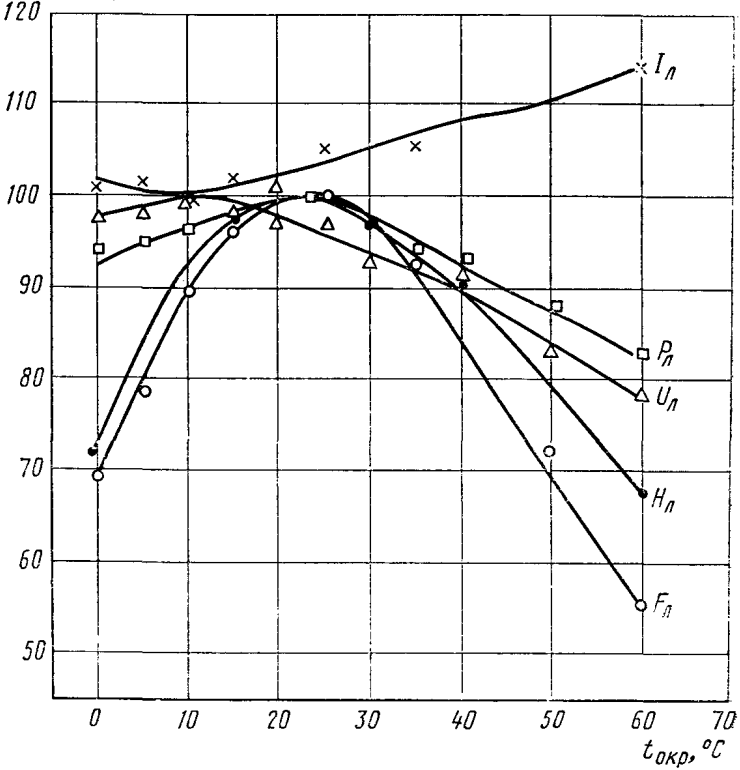
Зависимость параметров люминесцентных ламп мощностью 15 Вт от температуры окружающей среды
