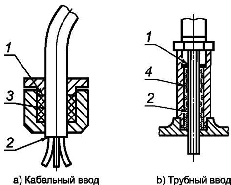
1 — место ввода кабеля; 2 — место разделки жил кабеля; 3 — уплотнительное кольцо; 4 — герметизирующий компаунд;
