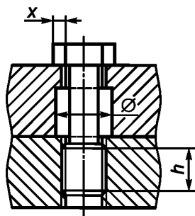
Рисунок 1 — Допуски и зазор для резьбовых крепежных деталей
