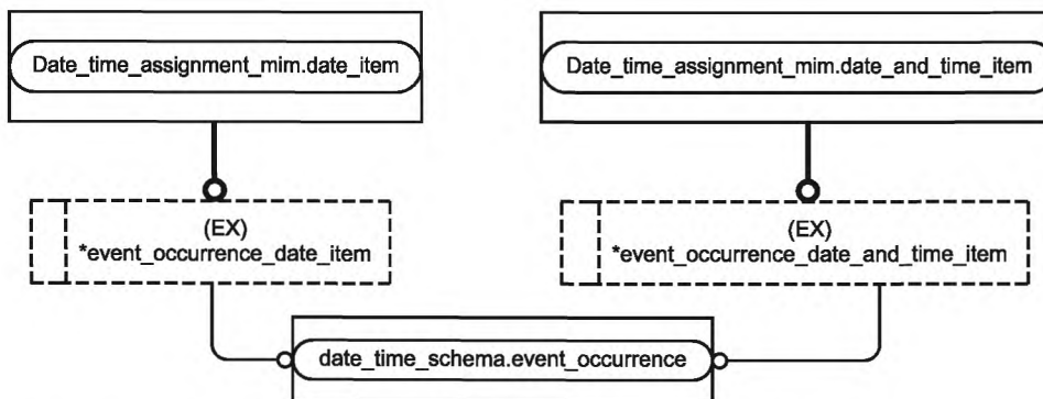
Рисунок D.2 — Представление ИММ на уровне объектов в формате EXPRESS-G (диаграмма 1 из 1)
