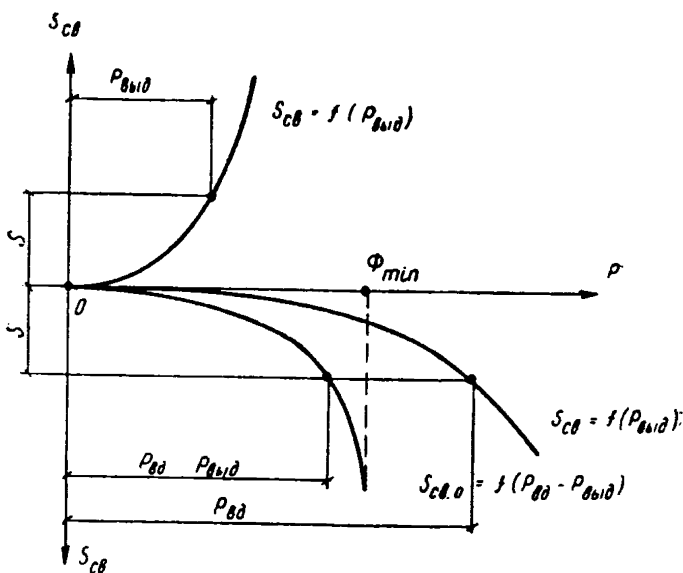
Рис. 2. Нахождение \Phi_{\min} по графику S_{св.о} = f(P_{вд} - P_{вйд})
