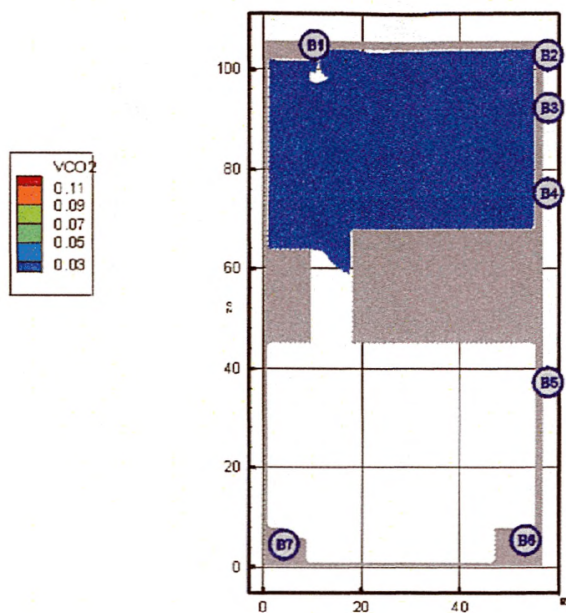
Рис. 32. Концентрация CO 2 (кг/м 3 ) в горизонтальном сечении на высоте 1,7 м от уровня пола в момент времени 300 с
