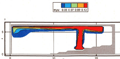
Рис. 85. Оптическая плотность дыма ( \text{Hn}/\text{м} ) в вертикальном сечении 1-1 в момент времени 130 с
