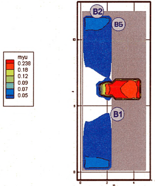
Рис. 154. Оптическая плотность дыма ( \text{Hп/м} ) в горизонтальном сечении на высоте 1,7 м от уровня пола в момент времени 100 с
