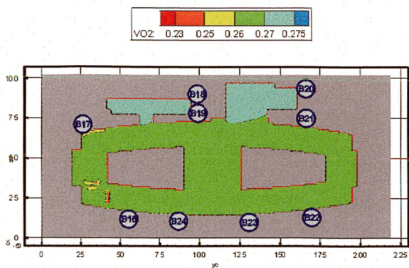
Рис. 71. Концентрация O_2 ( kg/m^3 ) в горизонтальном сечении на высоте 1,7 м от уровня пола третьего этажа в момент времени 1100 с
