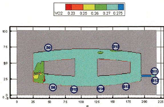
Рис. 70. Концентрация O_2 ( кг/м^3 ) в горизонтальном сечении на высоте 1,7 м от уровня пола второго этажа в момент времени 1100 с
