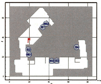
Рис. 126. Расчетная схема второго сценария развития пожара (горизонтальное сечение на высоте 1,7 м от уровня пола):
