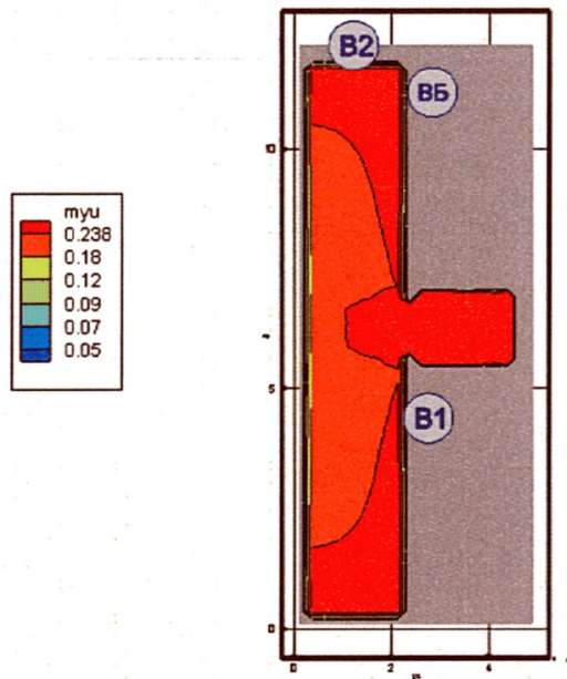
Рис. 155. Оптическая плотность дыма ( \text{Hп/м} ) в горизонтальном сечении на высоте 1,7 м от уровня пола в момент времени 160 с
