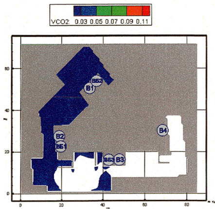
Рис. 149. Концентрация \text{CO}_2 ( \text{кг}/\text{м}^3 ) в горизонтальном сечении на высоте 1,7 м от уровня пола в момент времени 430 с
