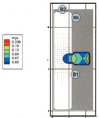
Рис. 179. Оптическая плотность дыма (Hп/м) в горизонтальном сечении на высоте 1,7 м от уровня пола в момент времени 60 с
