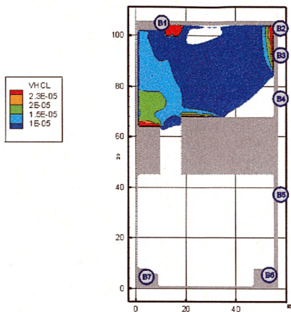
Рис. 36. Концентрация HCl ( \text{кг}/\text{м}^3 ) в горизонтальном сечении на высоте 1,7 м от уровня пола в момент времени 80 с
