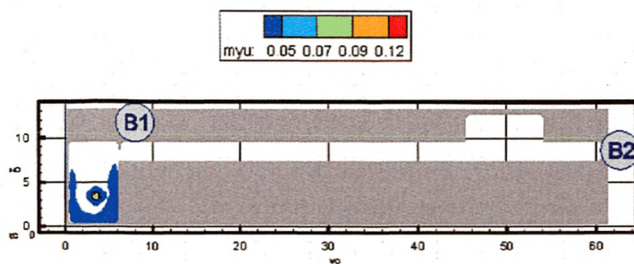
Рис. 99. Оптическая плотность дыма ( H_n/m ) в горизонтальном сечении на высоте 1,7 м от уровня пола в момент времени 60 с
