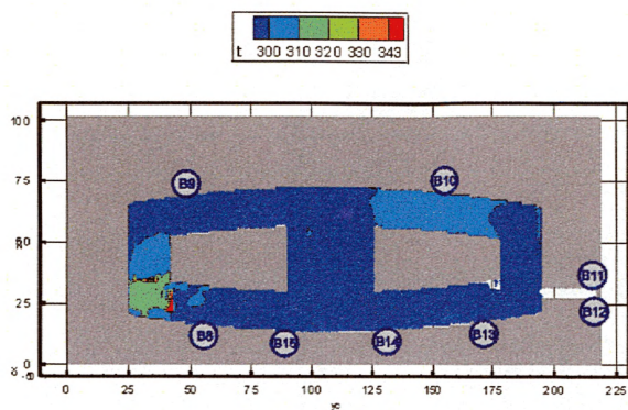
Рис. 61. Поля температуры (K) в горизонтальном сечении на высоте 1,7 м от уровня пола второго этажа в момент времени 1100 с
