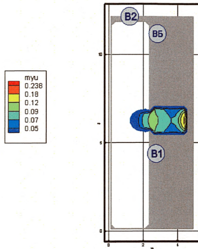
Рис. 153. Оптическая плотность дыма (Hn/m) в горизонтальном сечении на высоте 1,7 м от уровня пола в момент времени 60 с
