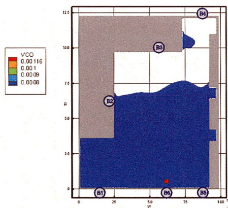
Рис. 44. Концентрация CO ( \text{кг}/\text{м}^3 ) в горизонтальном сечении на высоте 1,7 м от уровня пола в момент времени 1100 с
