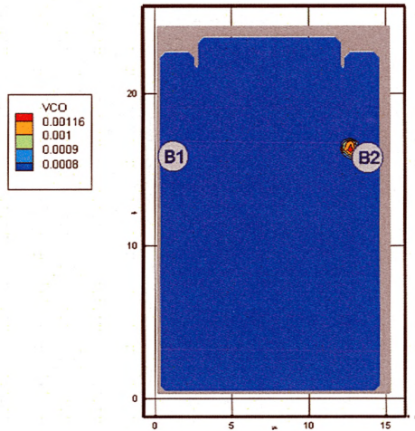
Рис. 91. Концентрация CO ( \text{кг}/\text{м}^3 ) в горизонтальном сечении на высоте 2,9 м от уровня пола в момент времени 410 с
