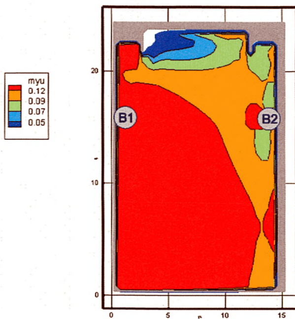
Рис. 87. Оптическая плотность дыма ( Hп/м ) в горизонтальном сечении на высоте 2,9 м от уровня пола в момент времени 230 с
