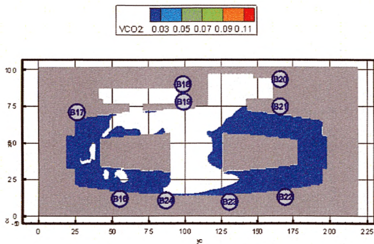
Рис. 66. Концентрация CO_2 ( кг/м^3 ) в горизонтальном сечении на высоте 1,7 м от уровня пола третьего этажа в момент времени 1100 с
