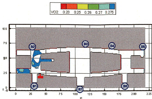
Рис. 69. Концентрация O_2 ( кг/м^3 ) в горизонтальном сечении на высоте 1,7 м от уровня пола первого этажа в момент времени 1100 с
