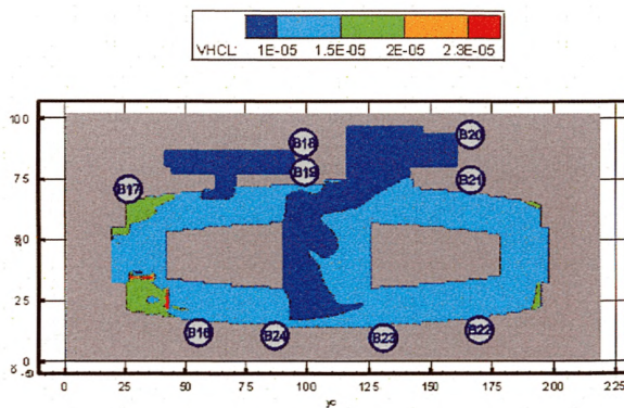
Рис. 72. Концентрация HCl ( kg/m^3 ) в горизонтальном сечении на высоте 1,7 м от уровня пола третьего этажа в момент времени 1100 с
