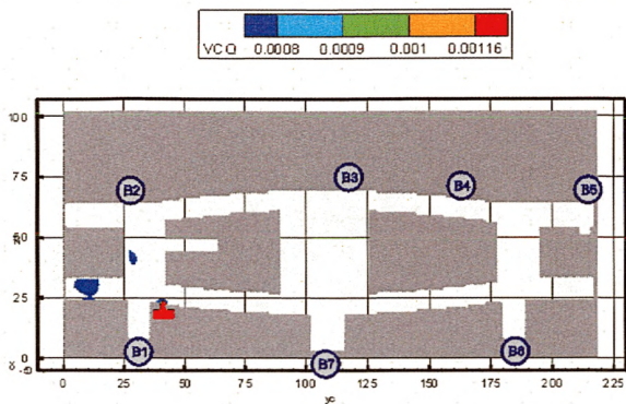
Рис. 63. Концентрация CO ( \text{кг}/\text{м}^3 ) в горизонтальном сечении на высоте 1,7 м от уровня пола первого этажа в момент времени 1100 с
