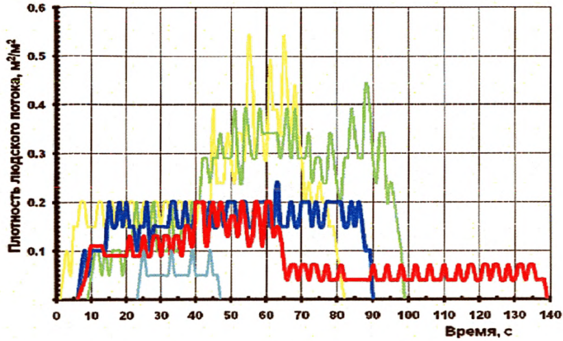
Рис. 121. Плотность людского потока на путях эвакуации (вариант 4):
