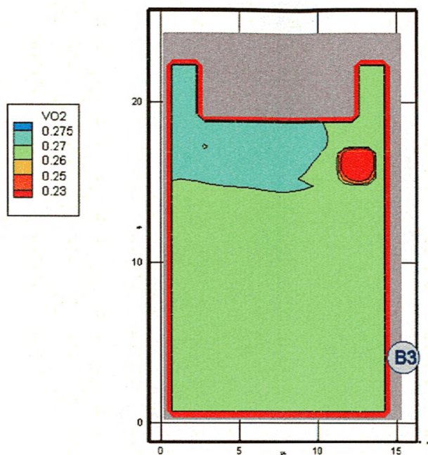
Рис. 96. Концентрация O_2 (кг/м 3 ) в горизонтальном сечении на высоте 1,7 м от уровня пола в момент времени 410 с
