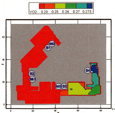
Рис. 150. Концентрация \text{O}_2 ( \text{кг}/\text{м}^3 ) в горизонтальном сечении на высоте 1,7 м от уровня пола в момент времени 430 с
