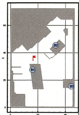
Рис. 125. Расчетная схема первого сценария развития пожара (горизонтальное сечение на высоте 1,7 м от уровня пола):
