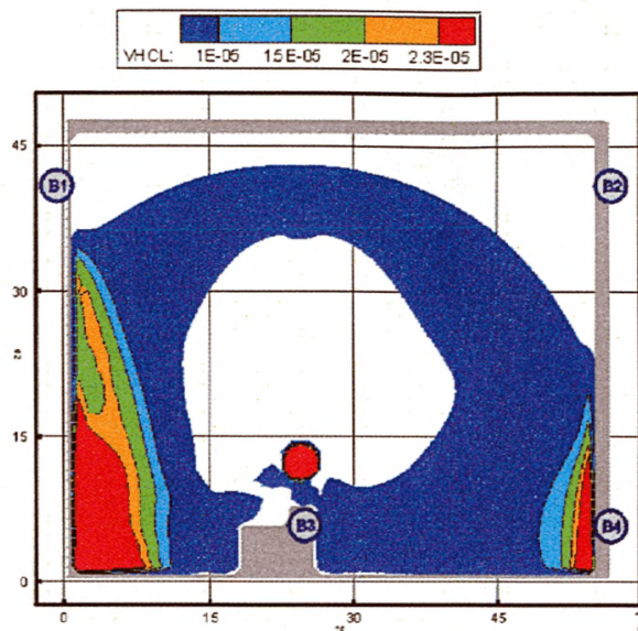
Рис. 20. Концентрация HCl ( \text{кг}/\text{м}^3 ) в горизонтальном сечении на высоте 1,7 м от уровня пола в момент времени 70 с
