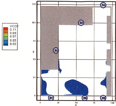
Рис. 45. Концентрация CO_2 ( кг/м^3 ) в горизонтальном сечении на высоте 1,7 м от уровня пола в момент времени 1100 с
