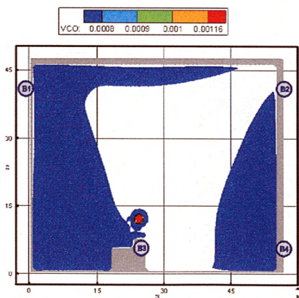
Рис. 17. Концентрация CO ( \text{кг}/\text{м}^3 ) в горизонтальном сечении на высоте 1,7 м от уровня пола в момент времени 100 с
