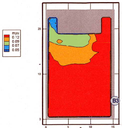
Рис. 88. Оптическая плотность дыма ( \mu /м) в горизонтальном сечении на высоте 1,7 м от уровня пола в момент времени 410 с
