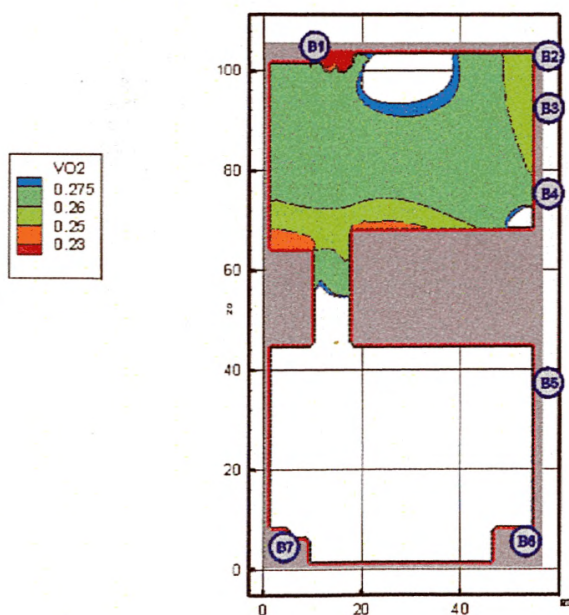
Рис. 33. Концентрация O 2 (кг/м 3 ) в горизонтальном сечении на высоте 1,7 м от уровня пола в момент времени 100 с
