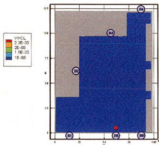
Рис. 47. Концентрация HCl ( \text{кг}/\text{м}^3 ) в горизонтальном сечении на высоте 1,7 м от уровня пола в момент времени 1100 с
