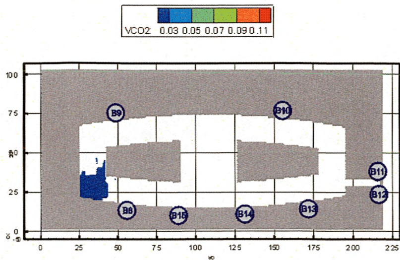
Рис. 67. Концентрация CO_2 ( кг/м^3 ) в горизонтальном сечении на высоте 1,7 м от уровня пола второго этажа в момент времени 1100 с
