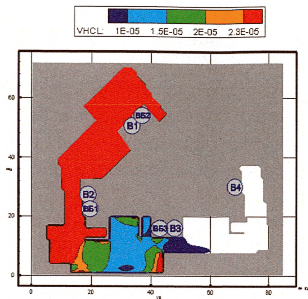
Рис. 151. Концентрация HCl ( \text{кг}/\text{м}^3 ) в горизонтальном сечении на высоте 1,7 м от уровня пола в момент времени 260 с
