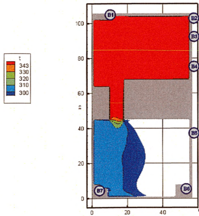
Рис. 30. Поля температуры (K) в горизонтальном сечении на высоте 1,7 м от уровня пола в момент времени 300 с
