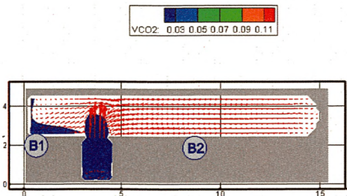
Рис. 167. Концентрация CO 2 ( \text{кг}/\text{м}^3 ) в горизонтальном сечении на высоте 1,7 м от уровня пола в момент времени 190 с
