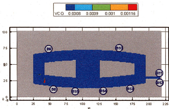
Рис. 64. Концентрация CO ( \text{кг}/\text{м}^3 ) в горизонтальном сечении на высоте 1,7 м от уровня пола второго этажа в момент времени 1100 с
