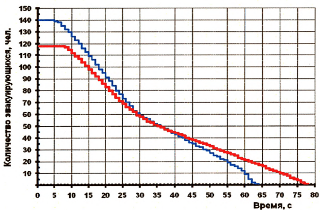
Рис. 114. Динамика эвакуации людей (вариант б):
