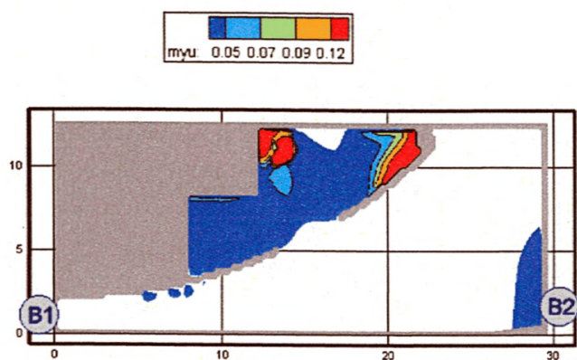
Рис. 76. Оптическая плотность дыма ( H_n/m ) в горизонтальном сечении на высоте 1,7 м от уровня пола в момент времени 150 с
