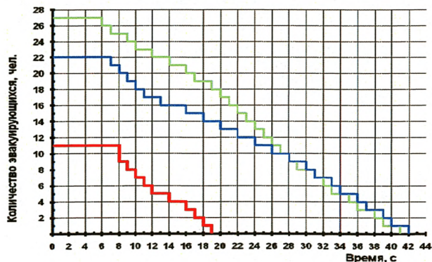
Рис. 110. Динамика эвакуации людей (вариант 1):
