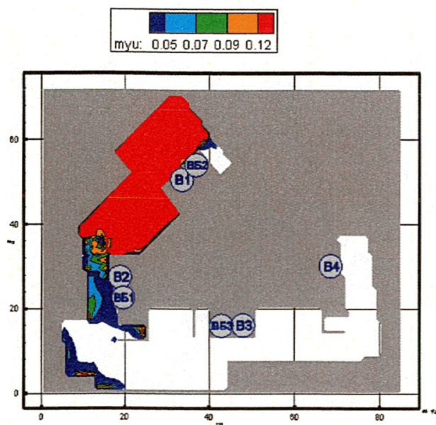
Рис. 141. Оптическая плотность дыма ( H_n/m ) в горизонтальном сечении на высоте 1,7 м от уровня пола в момент времени 120 с
