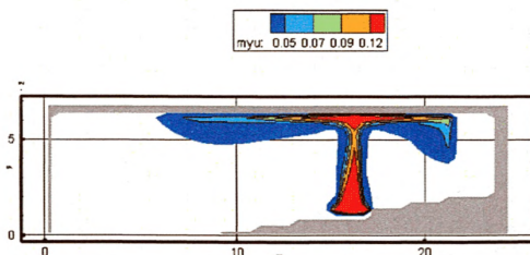
Рис. 84. Оптическая плотность дыма ( \text{Hn}/\text{м} ) в вертикальном сечении 1-1 в момент времени 80 с
