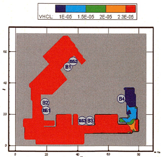
Рис. 152. Концентрация HCl ( \text{кг}/\text{м}^3 ) в горизонтальном сечении на высоте 1,7 м от уровня пола в момент времени 430 с
