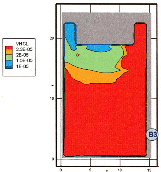
Рис. 97. Концентрация HCl (кг/м 3 ) в горизонтальном сечении на высоте 1,7 м от уровня пола в момент времени 410 с
