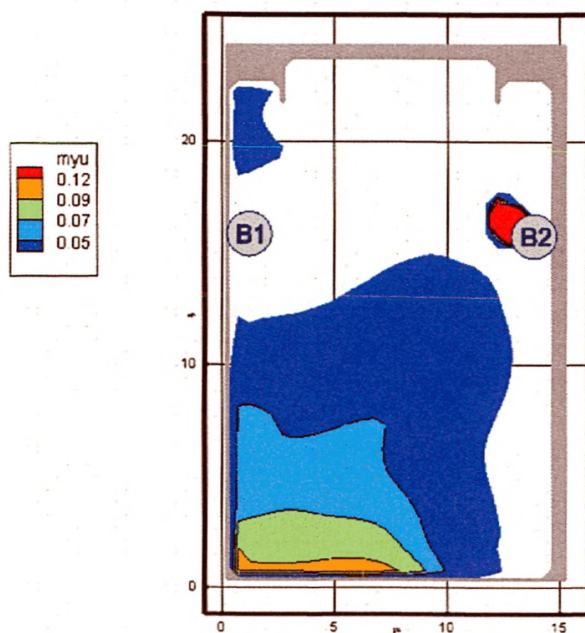
Рис. 86. Оптическая плотность дыма ( Hп/м ) в горизонтальном сечении на высоте 2,9 м от уровня пола в момент времени 170 с
