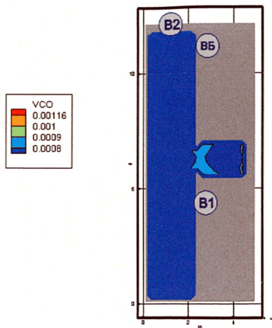
Рис. 157. Концентрация CO ( \text{кг}/\text{м}^3 ) в горизонтальном сечении на высоте 1,7 м от уровня пола в момент времени 160 с
