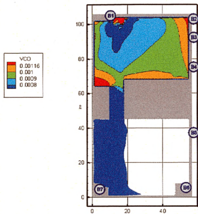
Рис. 31. Концентрация CO ( \text{кг}/\text{м}^3 ) в горизонтальном сечении на высоте 1,7 м от уровня пола в момент времени 300 с
