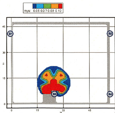
Рис. 11. Оптическая плотность дыма (Hn/м) в горизонтальном сечении на высоте 1,7 м от уровня пола в момент времени 20 с
