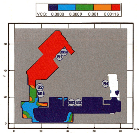
Рис. 148. Концентрация CO ( \text{кг}/\text{м}^3 ) в горизонтальном сечении на высоте 1,7 м от уровня пола в момент времени 430 с
