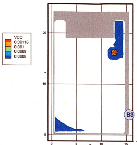
Рис. 92. Концентрация CO ( \text{кг}/\text{м}^3 ) в горизонтальном сечении на высоте 1,7 м от уровня пола в момент времени 410 с
