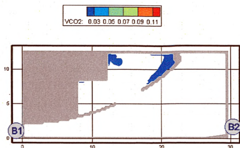
Рис. 81. Концентрация CO_2 ( кг/м^3 ) в горизонтальном сечении на высоте 1,7 м от уровня пола в момент времени 220 с
