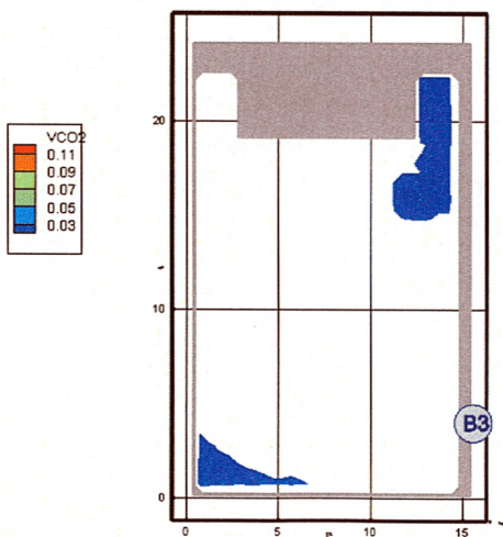
Рис. 93. Концентрация CO₂ ( \text{кг}/\text{м}^3 ) в горизонтальном сечении на высоте 1,7 м от уровня пола в момент времени 410 с
