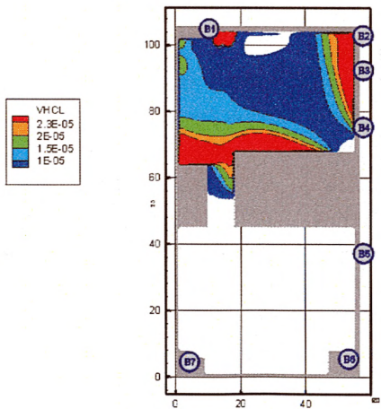
Рис. 37. Концентрация HCl ( \text{кг}/\text{м}^3 ) в горизонтальном сечении на высоте 1,7 м от уровня пола в момент времени 100 с
