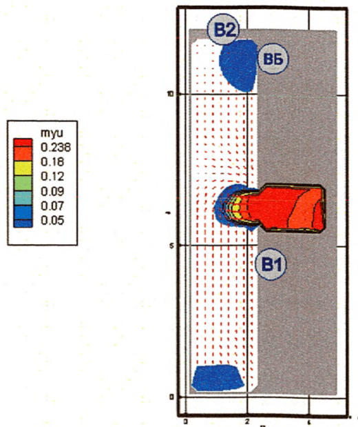
Рис. 180. Оптическая плотность дыма (Hn/м) в горизонтальном сечении на высоте 1,7 м от уровня пола в момент времени 100 с
