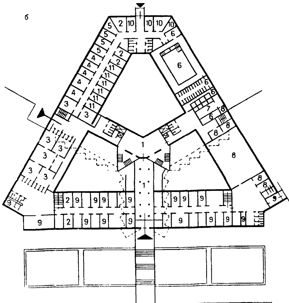
Рис. 1.9. Санаторий «Родербиркен» на 252 места в Ляйхлинае, Австрия
