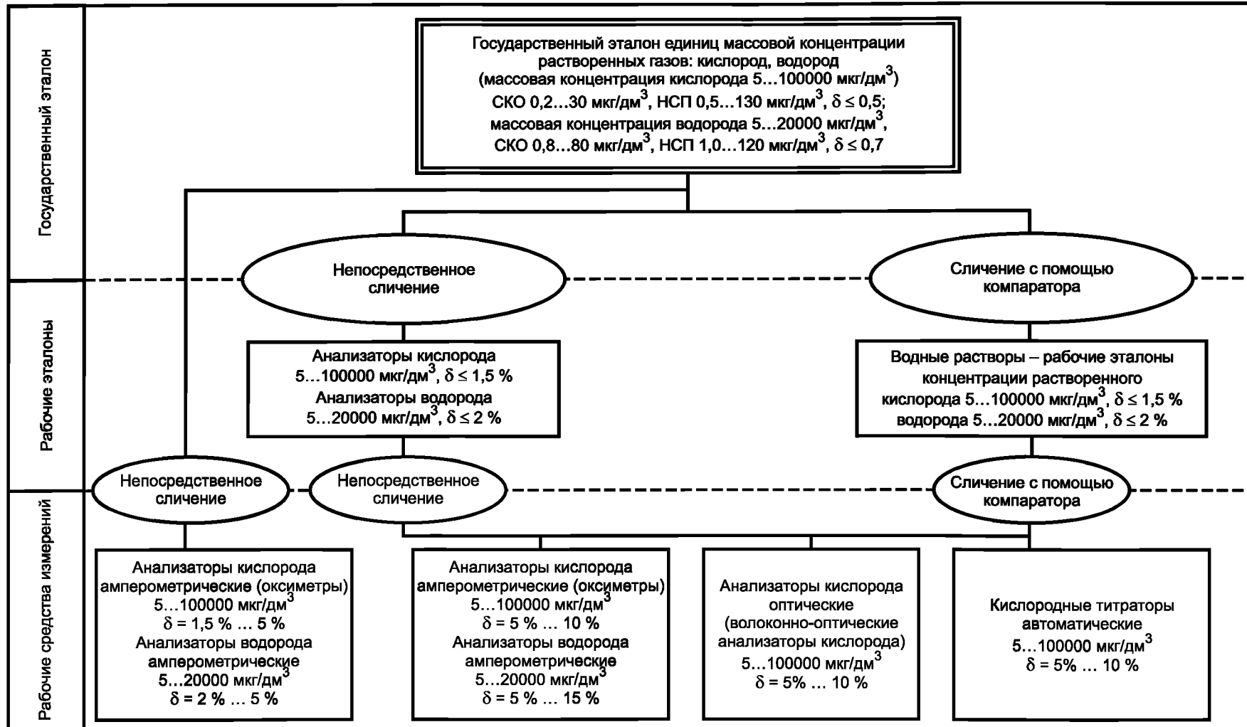
Рисунок А.1 – Государственная поверочная схема
