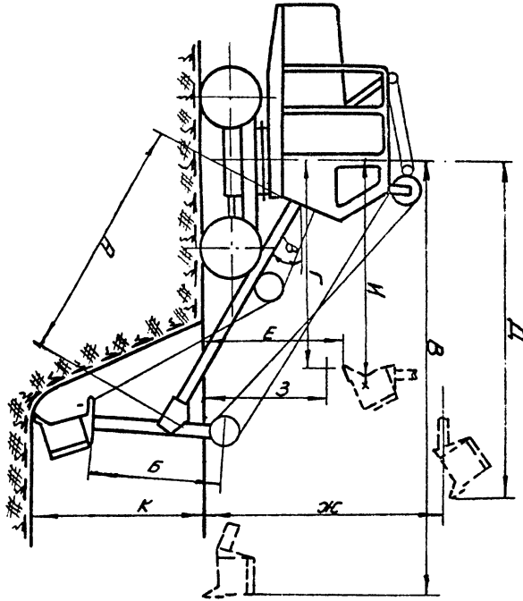
Техническая характеристика экскаватора Э-302, оборудованного обратной лопатой.
