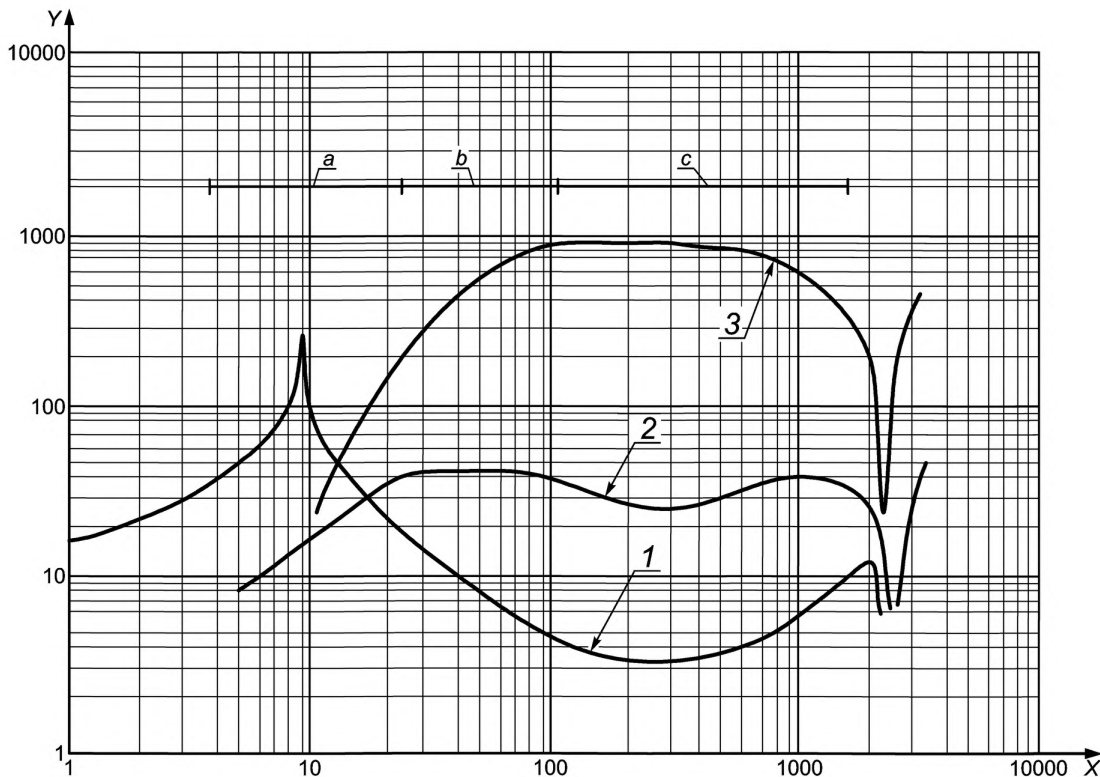
X — частота, Гц; Y — импеданс (кривая 1), ток (кривая 2) или напряжение (кривая 3) в условных единицах; a — область постоянного перемещения; b — область постоянной скорости; c — область постоянного ускорения
