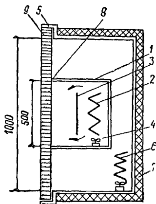
Рис. 9. Схема прибора для испытания термического сопротивления сотопласта
