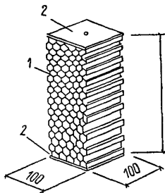
Рис. 11. Форма и размеры образца для определения коэффициента линейного теплового расширения
