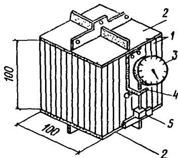
Рис. 6. Внешний вид составного образца для определения модуля упругости при растяжении сотопласта
