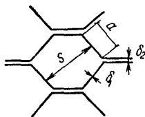
Рис. 8. Параметры сотовой структуры
