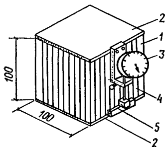
Рис. 5. Внешний вид составного образца для определения модуля упругости при сжатии сотовпласта
