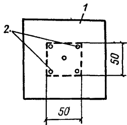
Рис. 10. Схема размещения термопар на поверхности образца для испытания
