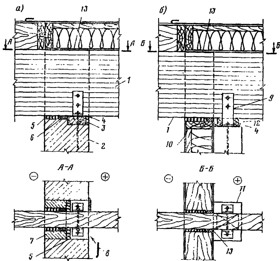
Рис. 2. Устройство узла сопряжения несущей ДКК
