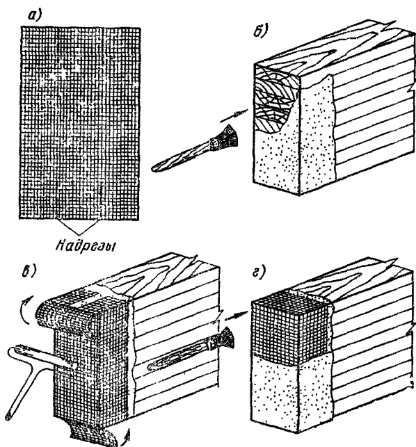
Рис. 16. Устройство армированного покрытия
