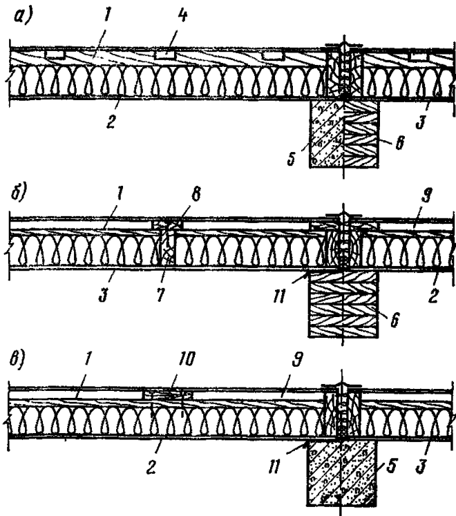
Рис. 10. Вентилирование стеновых панелей и примыкание их к стойкам
