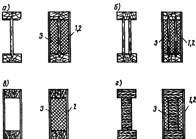
Рис. 13. Способы повышения огнестойкости несущих ДКК
