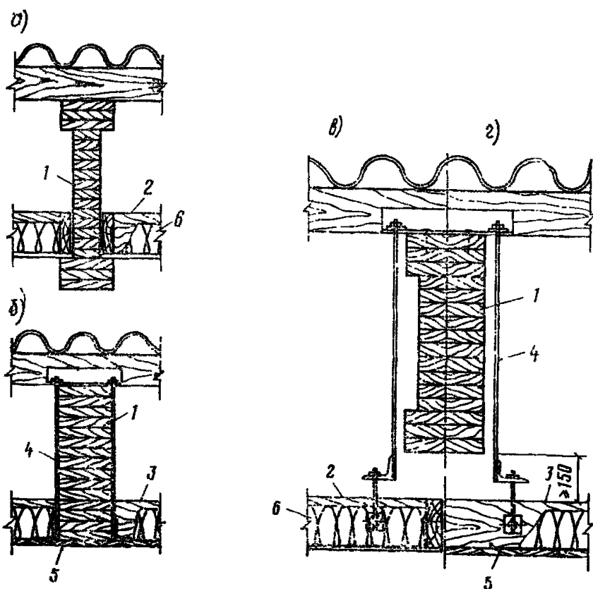
Рис. 6. Устройство подвесного потолка
