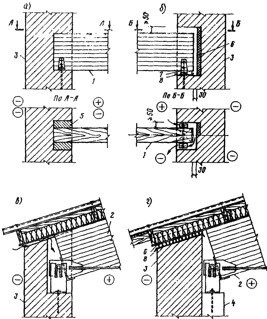
Рис. 5. Опирание несущих ДКК на наружные стены с выделкой гнезд
