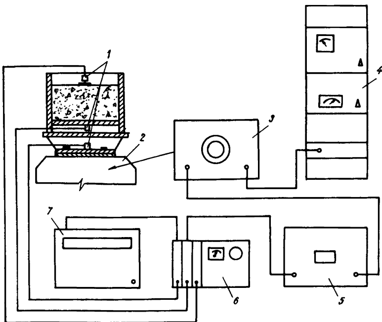
Рис.10. Схема измерительного тракта для исследования характеристик системы вибромашина-форма-бетонная смесь
