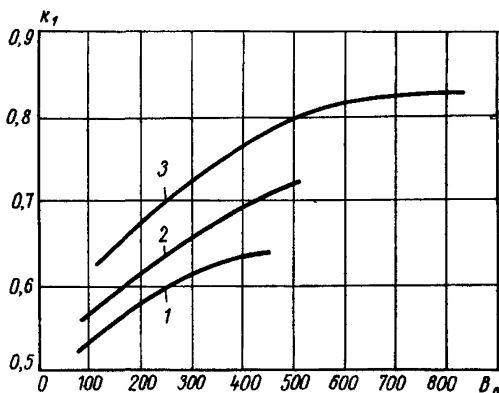
Рис.3. Зависимость коэффициента частичного заземления K_1 от параметров ячейки и рамы из полосовой стали. Значения B_0 увеличены в 10^8 раз.
