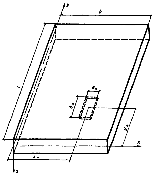
Рис.9. Схема обозначений поддона с подмагнитными плитами как плиты с сосредоточенными массами
