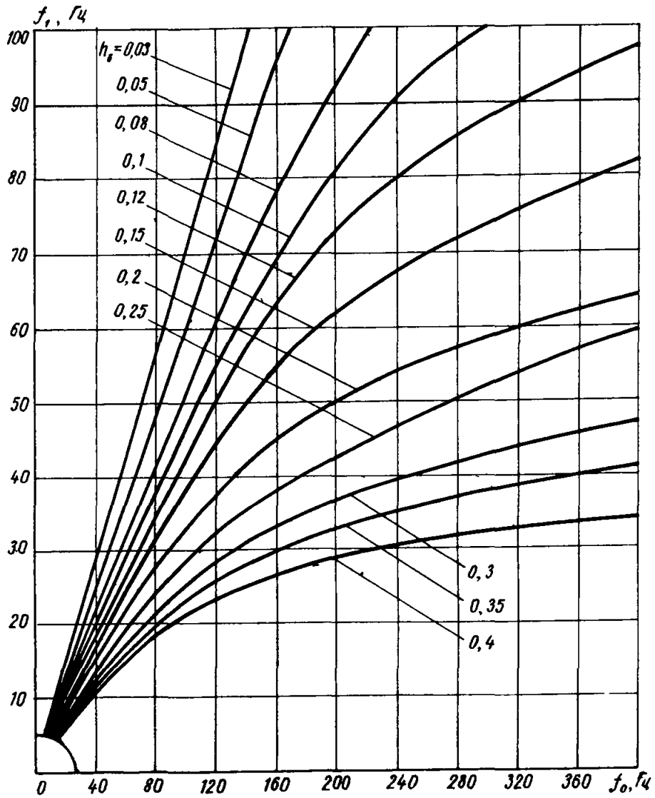
Рис.7. График для определения частоты основного тона колебаний обшивки со смесью f_1 в зависимости от частоты f_0 и высоты смеси h_s .
