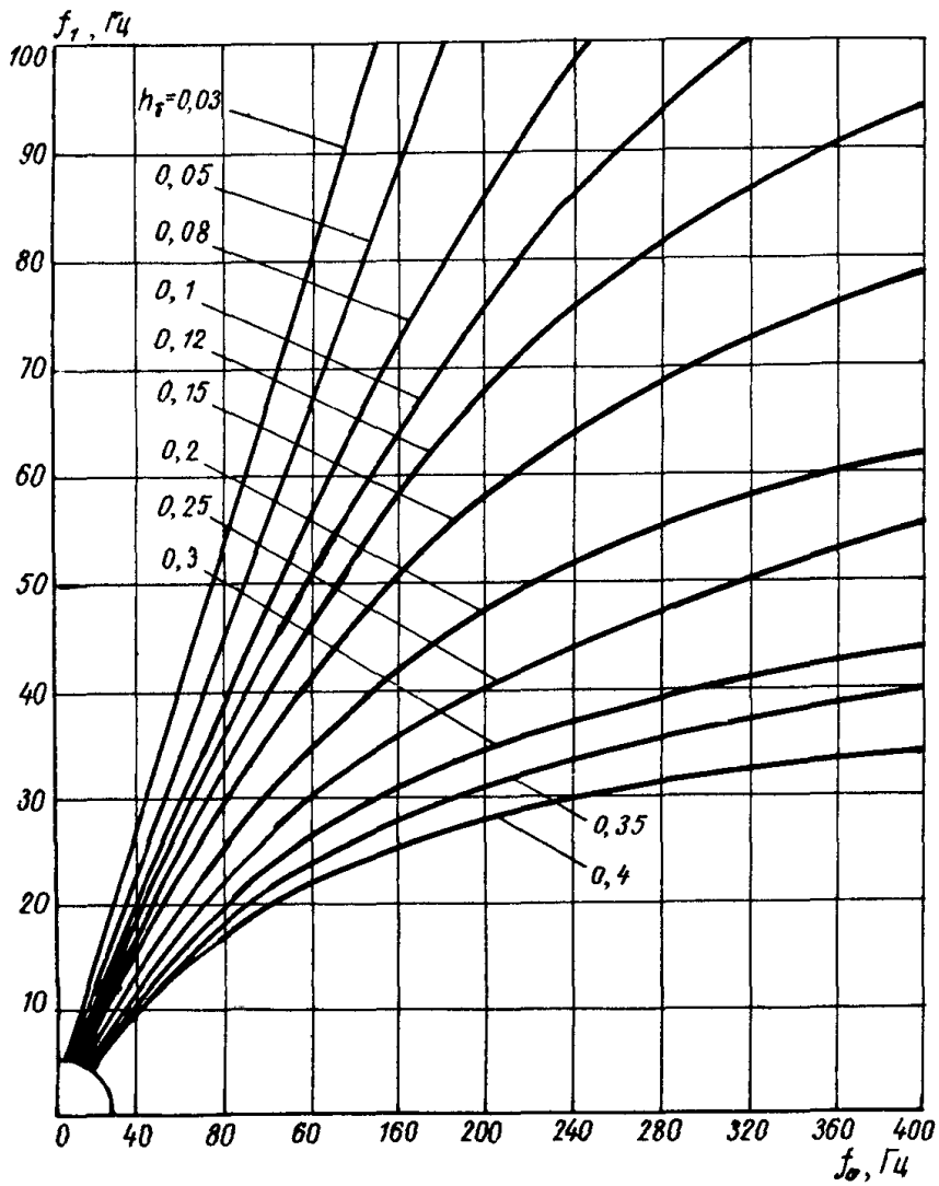
Рис.6. График для определения частоты основного тона колебаний обшивки со смесью f_1 в зависимости от частоты f_0 и высоты смеси h_f .
