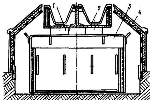
Рис. 4. Виброплощадка с формой и звукоизолирующими ограждениями
