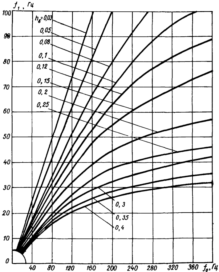
Рис.5. График для определения частоты основного тона колебаний ошывки со смесью f_1 в зависимости от частоты f_0 и высоты смеси h_g .
