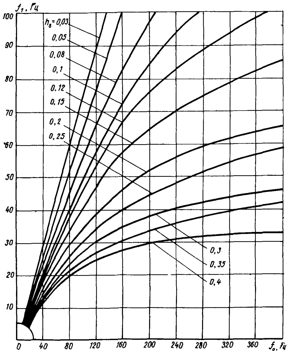
Рис.8. График для определения частоты основного тона колебаний обшивки со смесью f_1 в зависимости от частоты f_0 и высоты смеси h_\delta .
