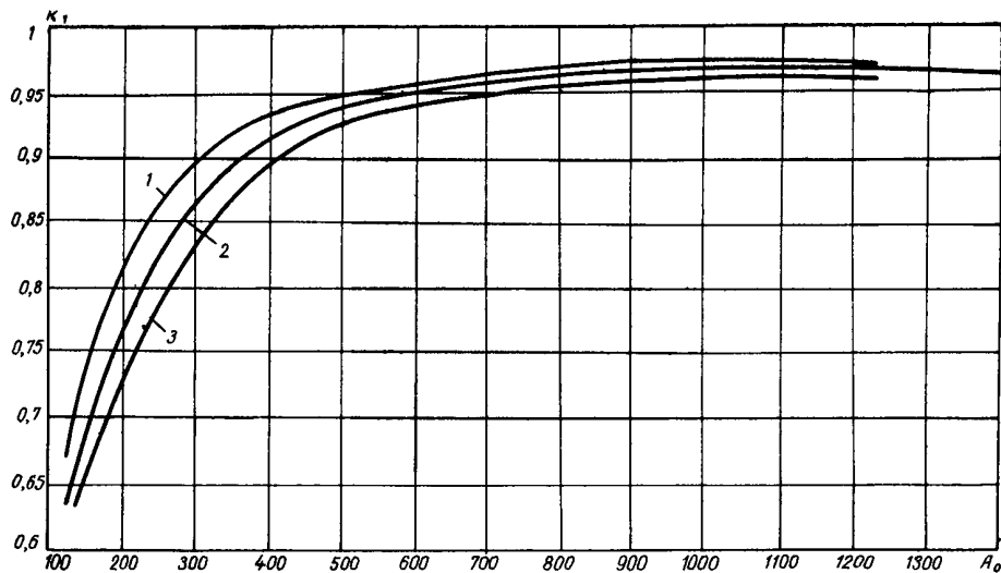
Рис.2. Зависимость коэффициента частичного заземления \kappa_1 от параметров ячейки и рамы (из одинарных швеллеров). Значения A_0 увеличены в 10^8 раз 1 - a/v, = 1 ; 2 - a/v, = 1,5 ; 3 - a/v, = 2
