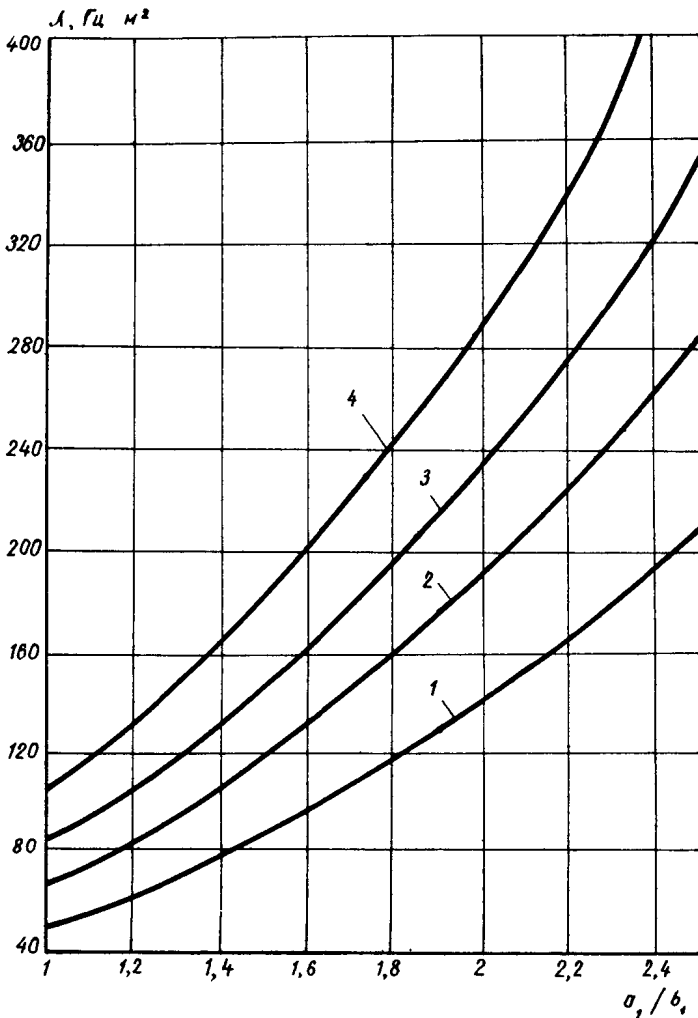
Рис. I. Зависимость частоты основного тона колебаний заземленной по контуру прямоугольной пластины от отношения сторон ячейки и толщины обшивки.
