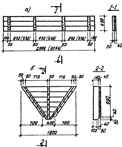
Рис.7 Фиты опалубки
