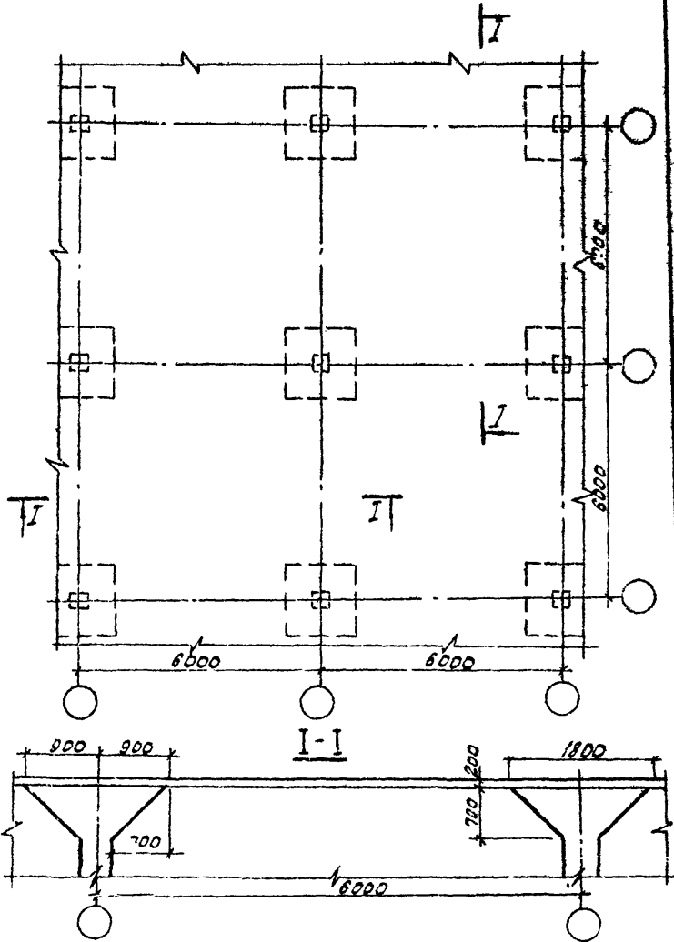
Рис. I Конструкция безбалочного перекрытия
