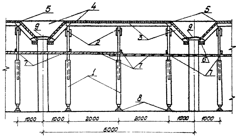
Рис. 4 Разрез К-К
