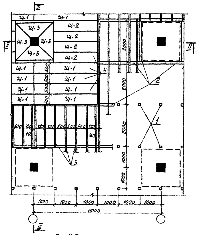
Рис.2 Конструкция опалубки в плане
