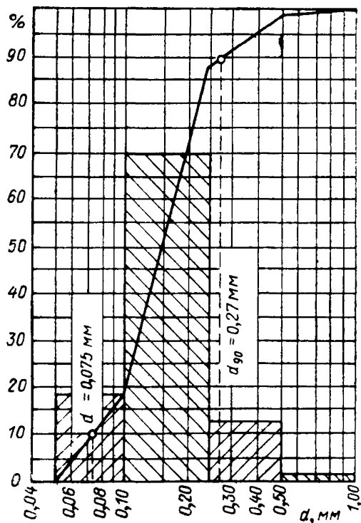
Рис. 10. Кривая гранулометрического состава и гистограмма фракций однофазного грунта.
