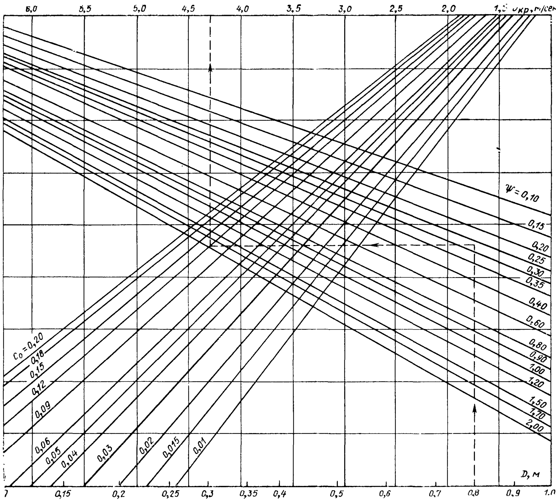
Рис. 3. Номограмма для расчета v_{кр} по формуле v_{кр} = 8,3 \sqrt[3]{D} \sqrt[6]{\psi_{ср} \epsilon_0}
