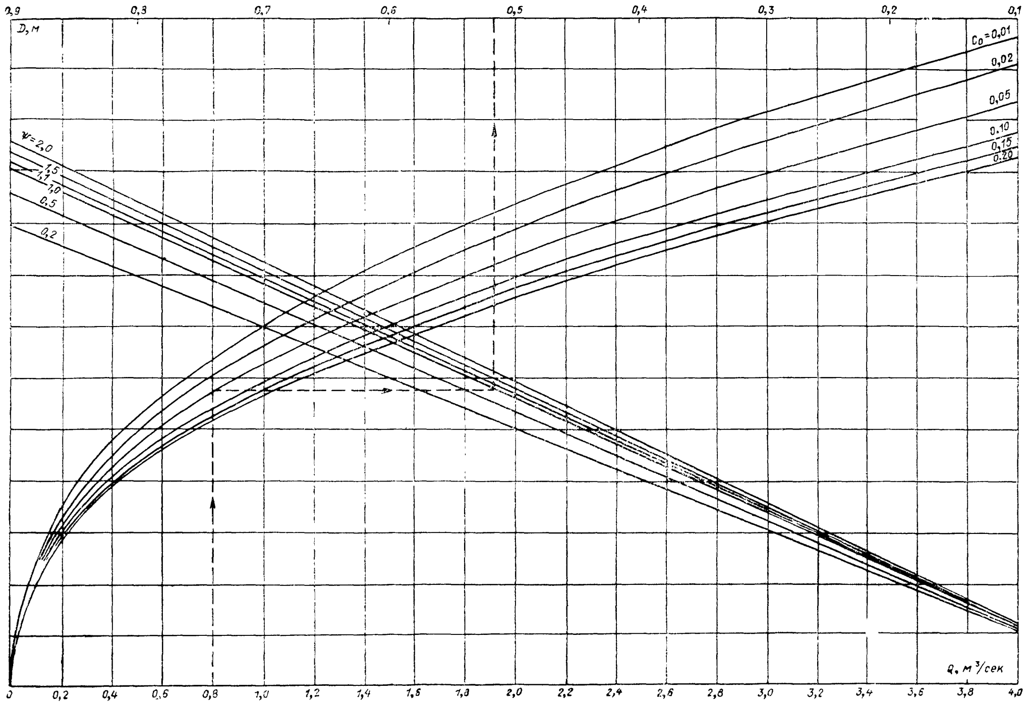
Рис. 8. Номограмма для определения диаметра трубопровода D
